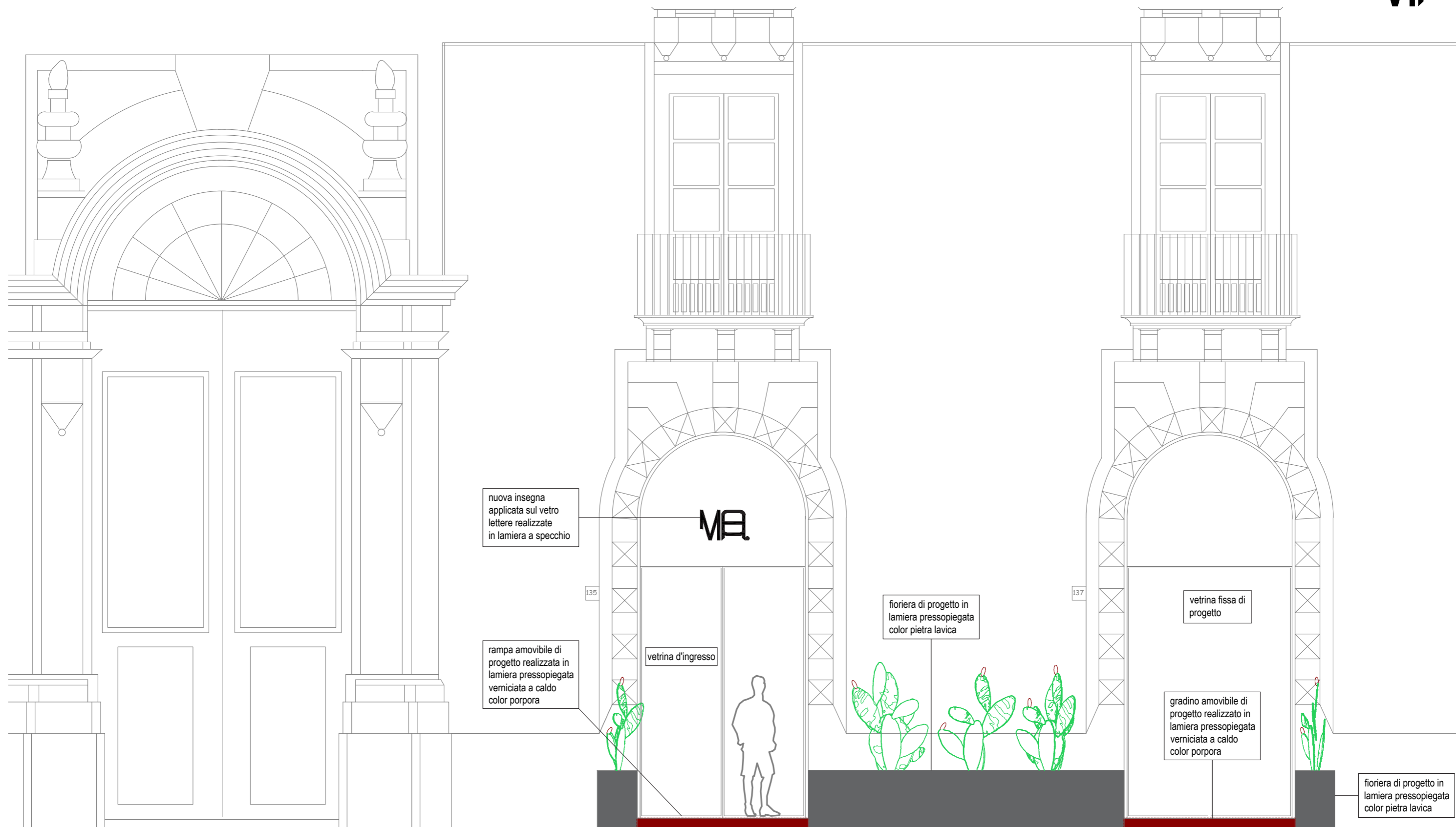
PROSPETTO ESTERNO DI PROGETTO
