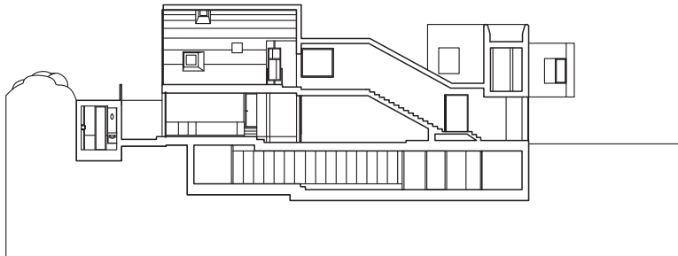
COUPE A-A
