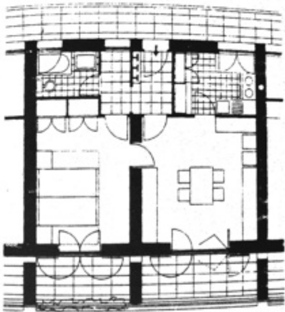
Fig. 13. I. Diotallevi e F. Marescotti, Villaggio per le maestranze del lanificio "Fila" a Cossato (1943): pianta alloggio tipo.
