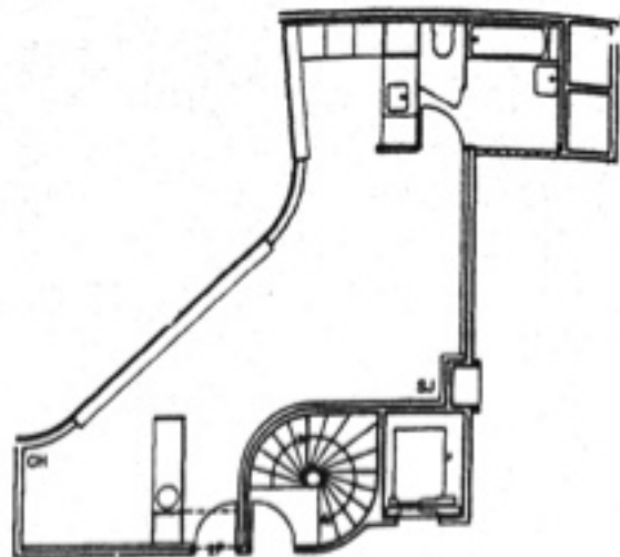
Fig. 8. B. Dolle e C. Labbé, Alloggio monostanza per impiegati delle Poste in rue de la Reine-Blanche a Parigi.
