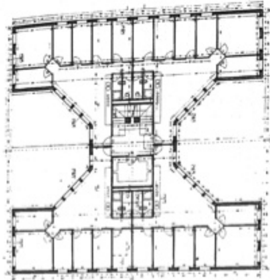
Fig. 5. L. Vacchini, "Casa Maria" - Ostello per operai stagionali a Dietlikon (ZH): pianta piano tipo (quattro alloggi).
