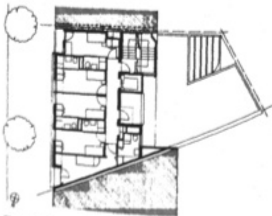
Fig. 7. O. Chaslin, "Résidence meublée" in rue des Pyrénées a Parigi: pianta piano tipo.
