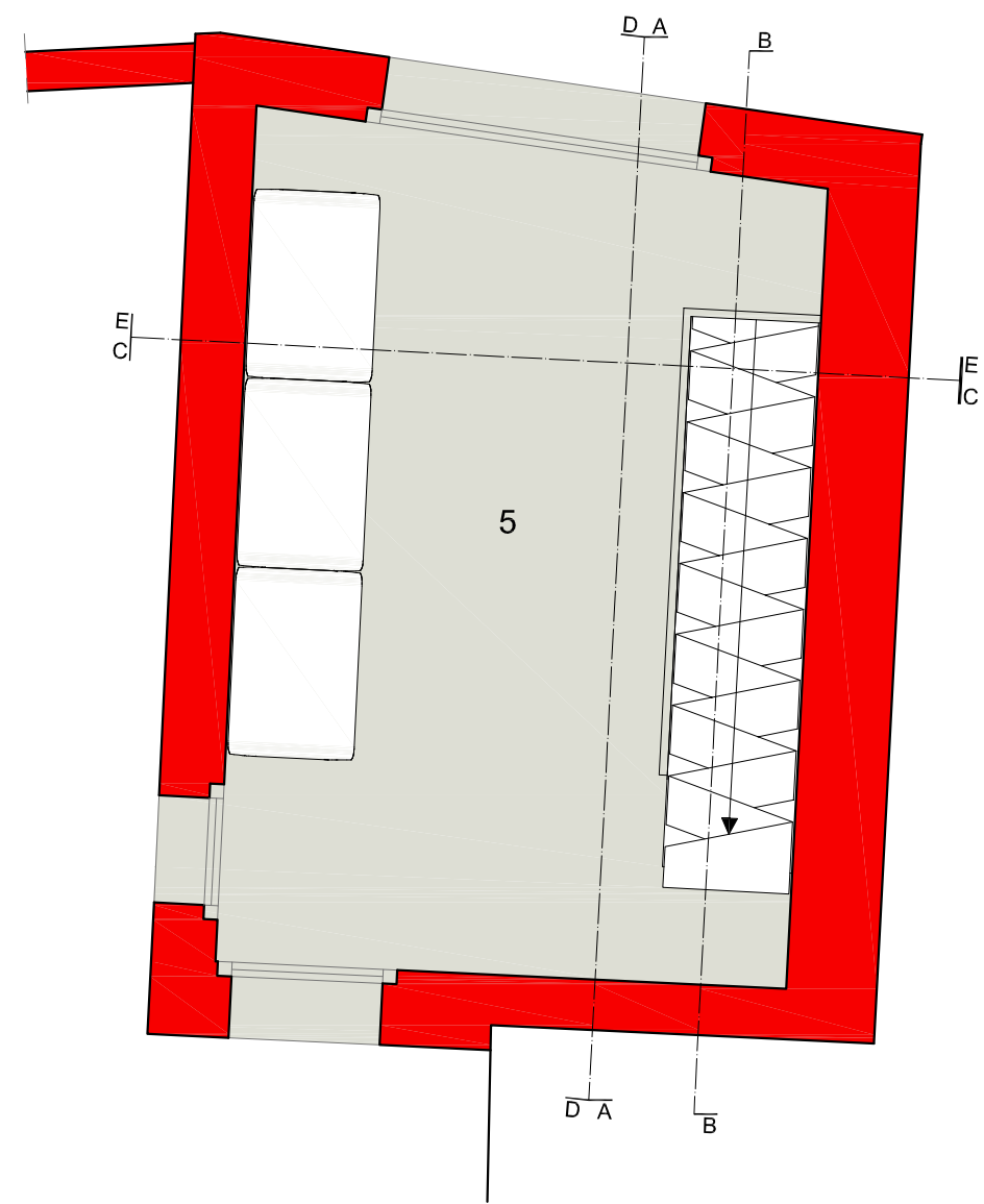
PIANO PRIMO
