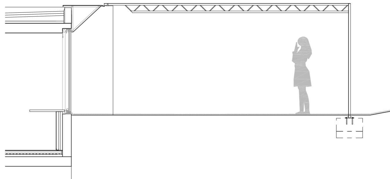
PÈRGOLA - ALÇAT LATERAL
