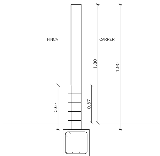
TANCA CARRER - SECCIÓ
