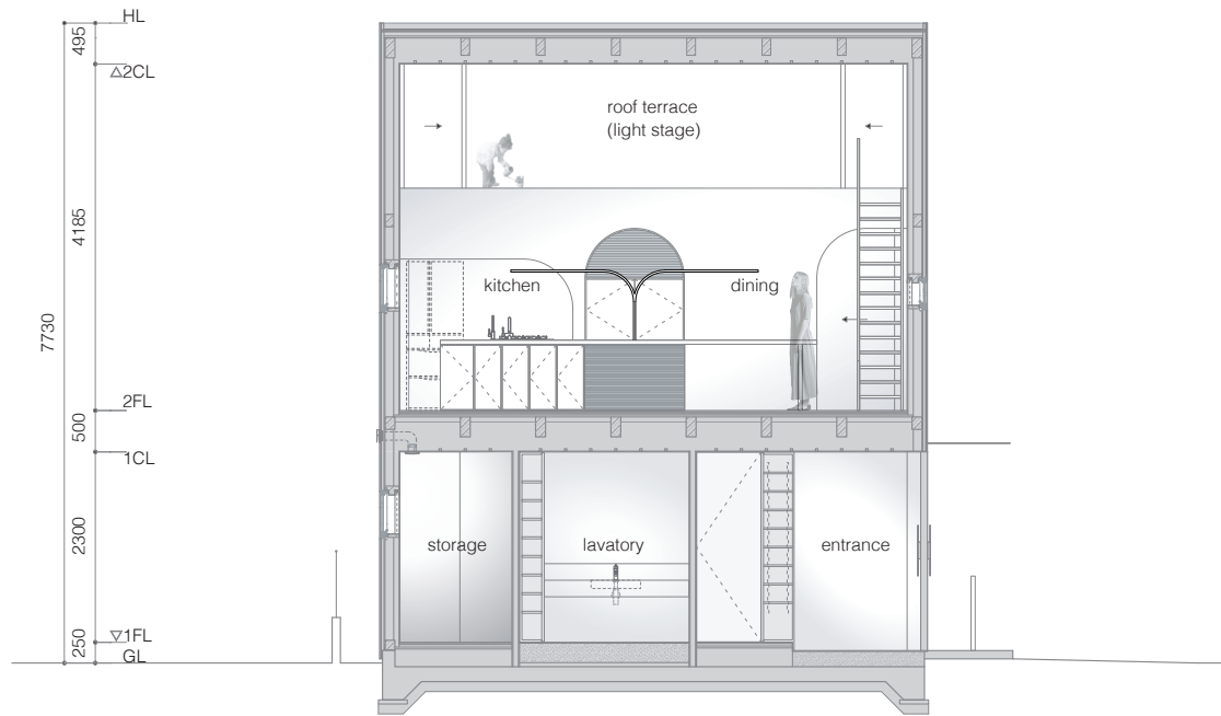
section 02 1:100
