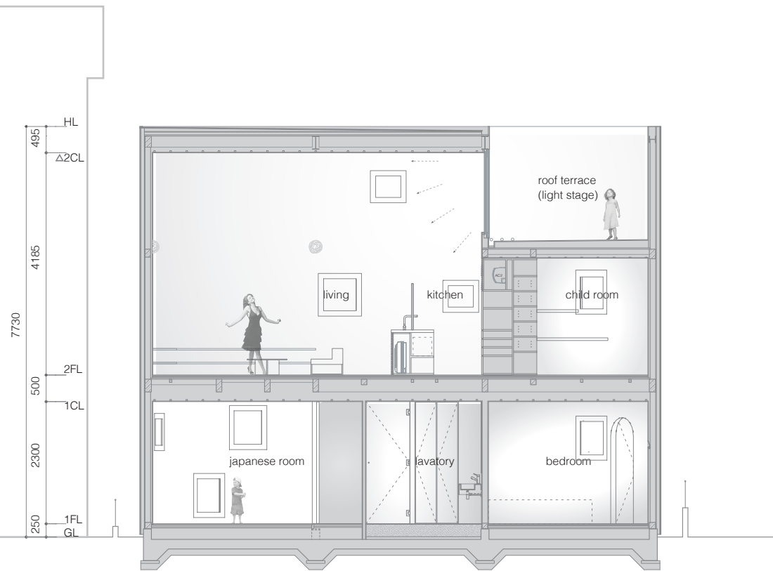
section 01 1:100
