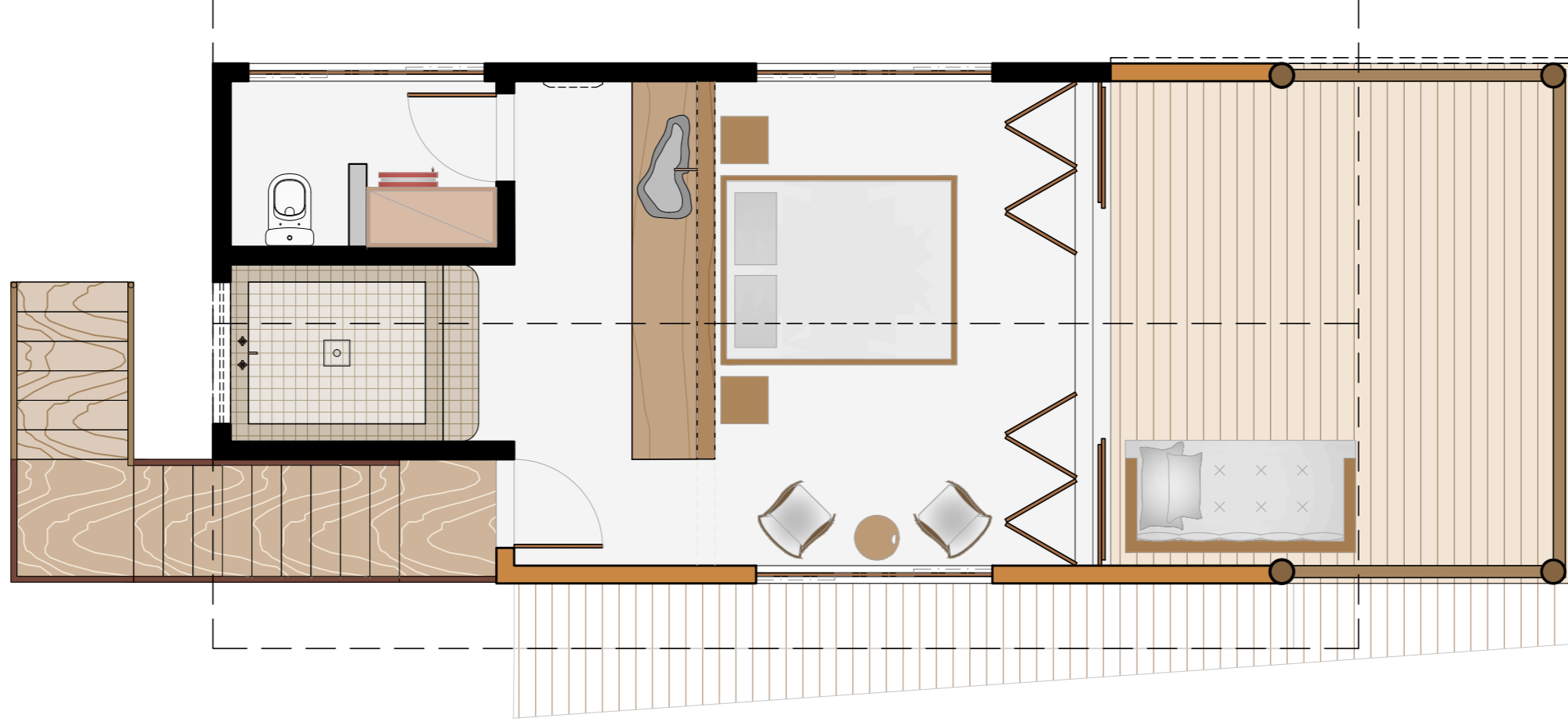
POUSADA HAYÔ | 2º PAV. SUÍTE 2 | PLANTA LAYOUT
