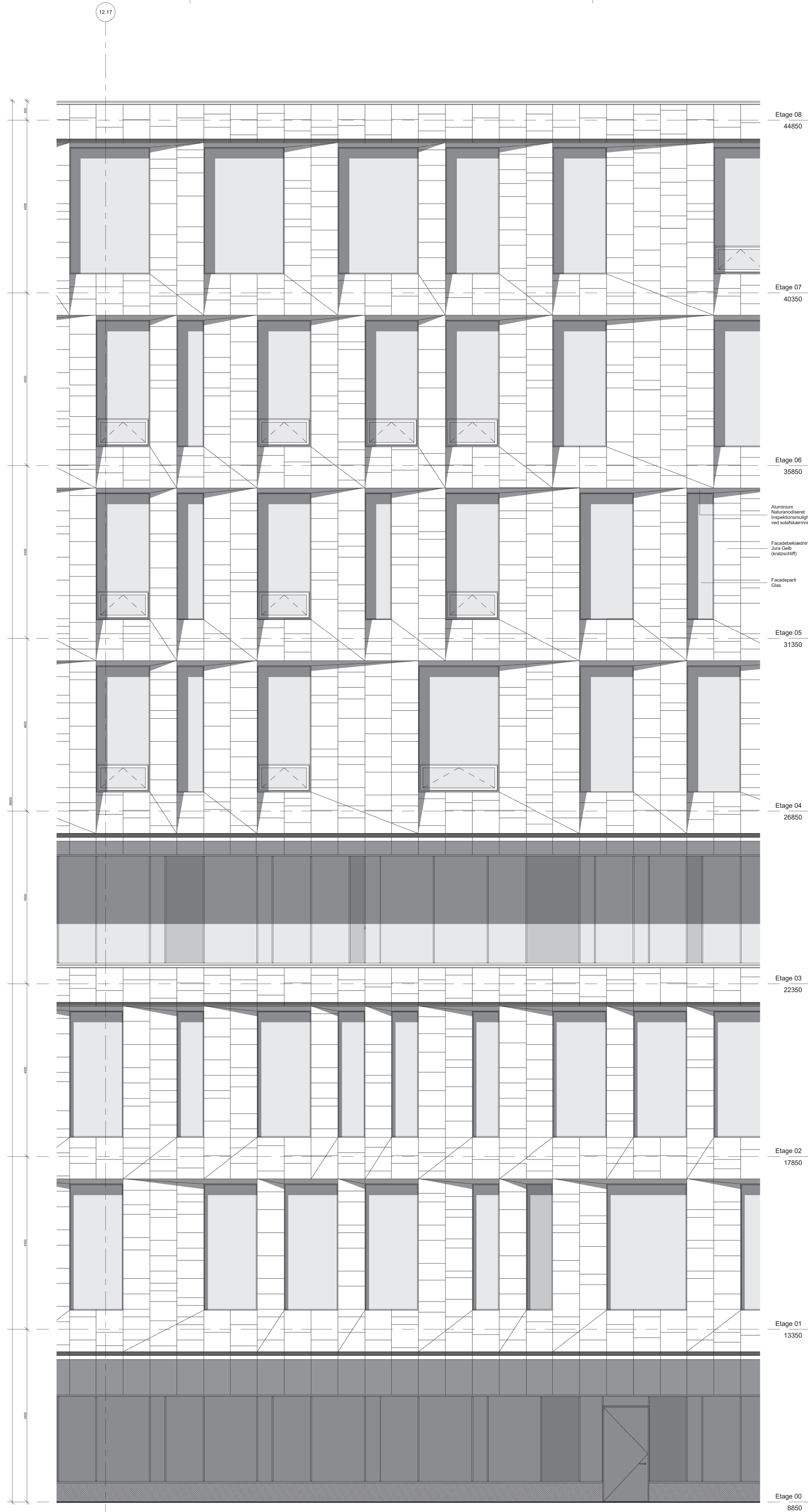
Facadeudsnit nordfacade 1:50
