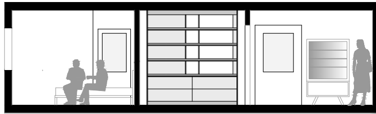
1_LONGITUDINAL SECTION
