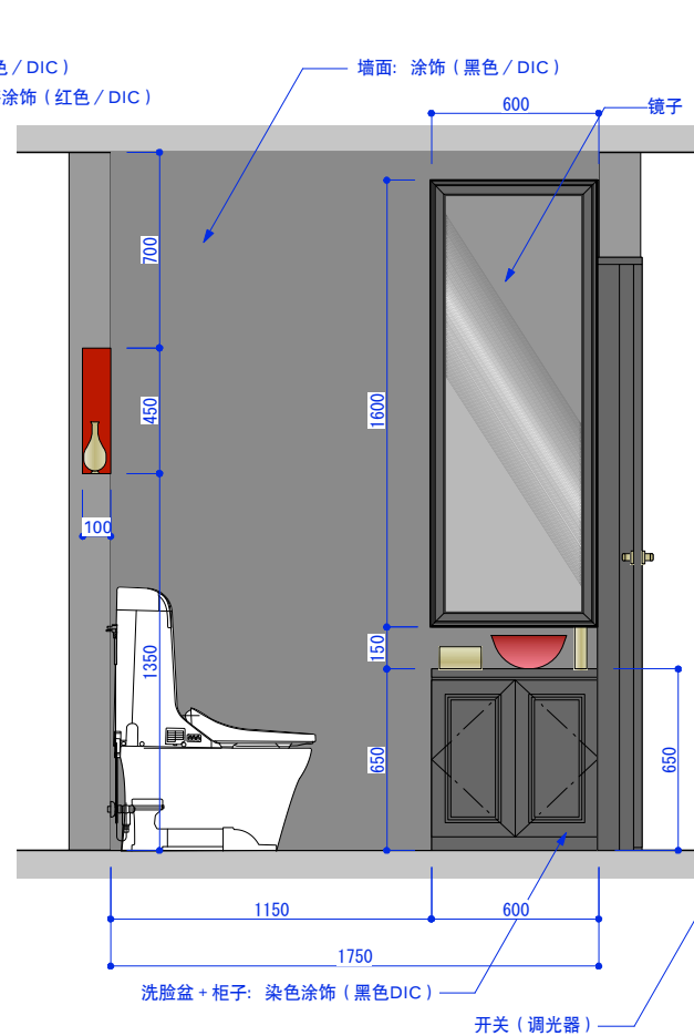
立面展开图K
