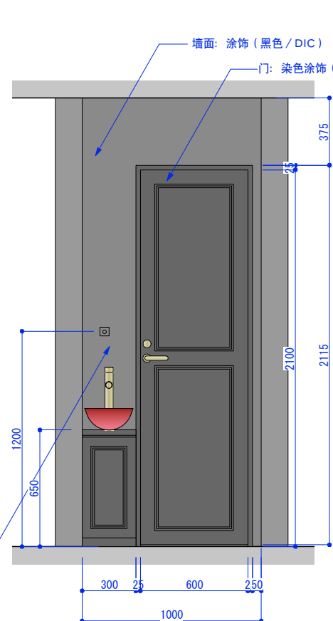
立面展开图L
