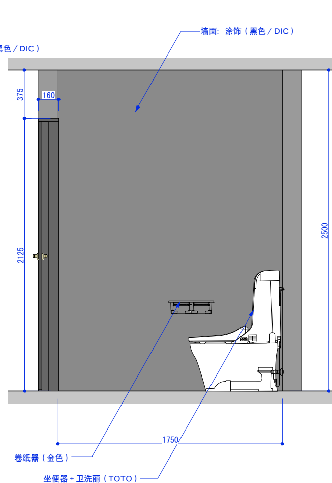
立面展开图M
