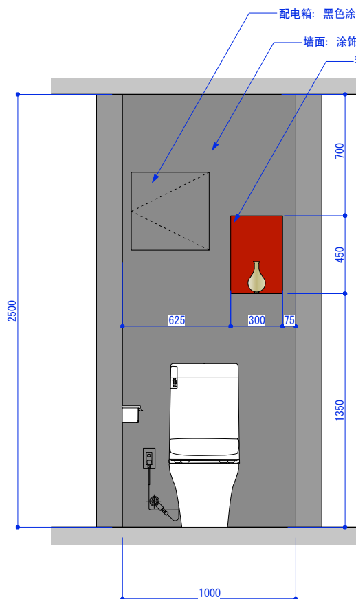
立面展开图J
