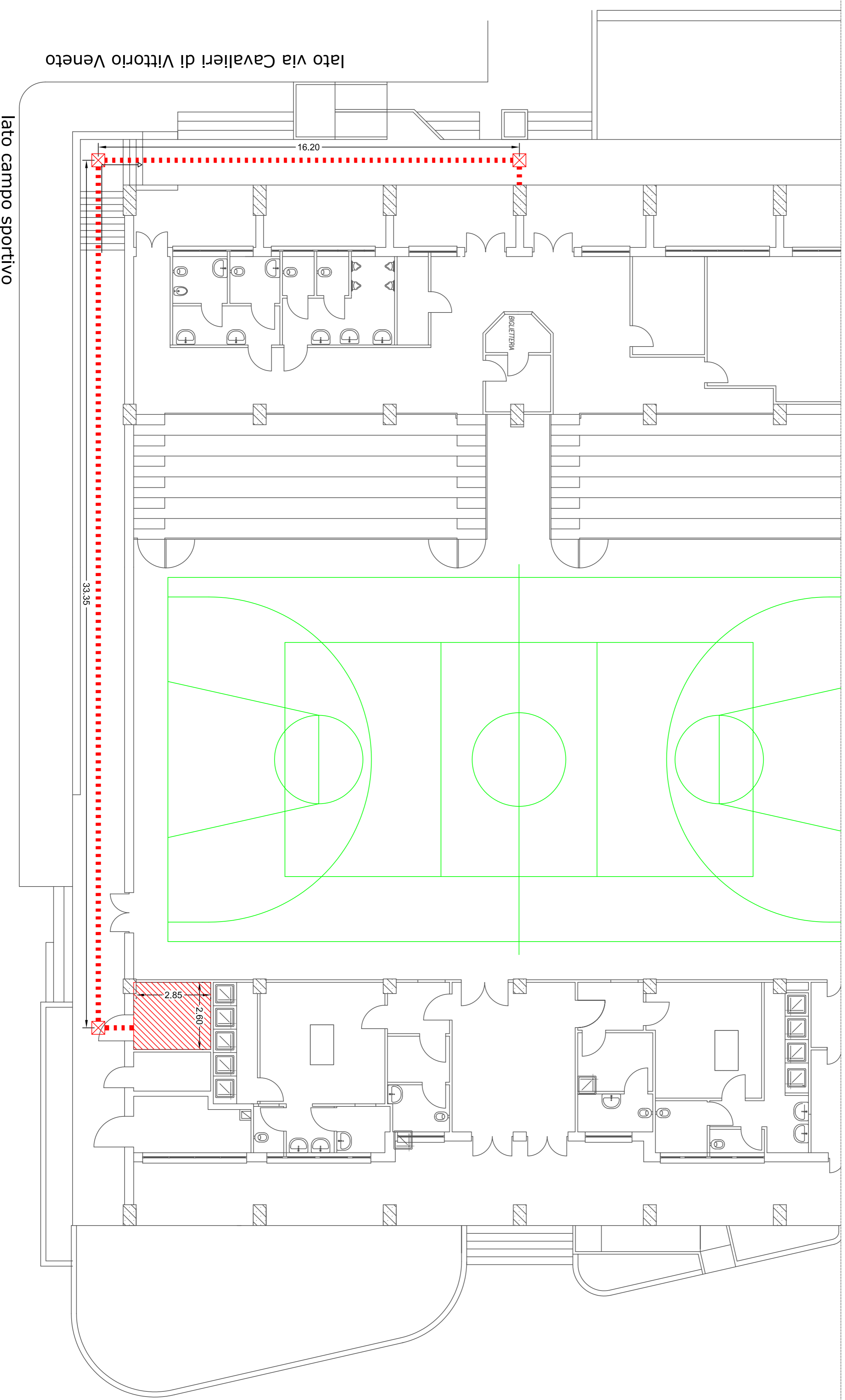
planimetria locali tecnici (piano terra)
