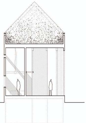
SECCIÓN DD'
