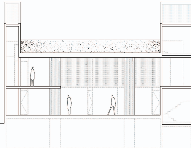
SECCIÓN CC'
