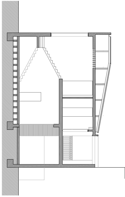
seziona X-X: stato di fatto - scala 1:100
