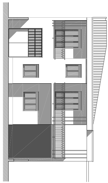
prospetto OVEST: stato di fatto - scala 1:100
