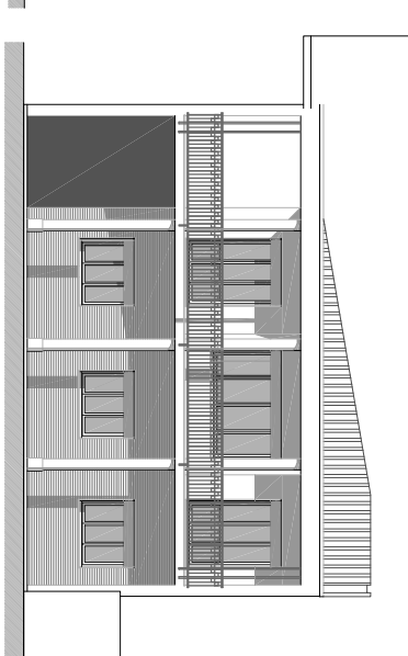
prospetto EST: stato di fatto - scala 1:100
