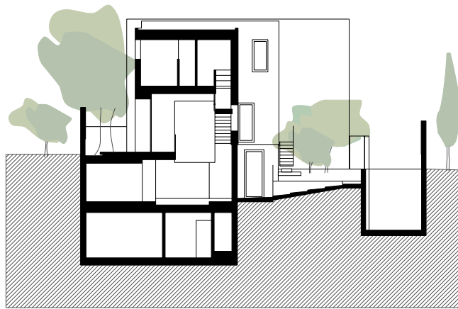
Sección transversal
