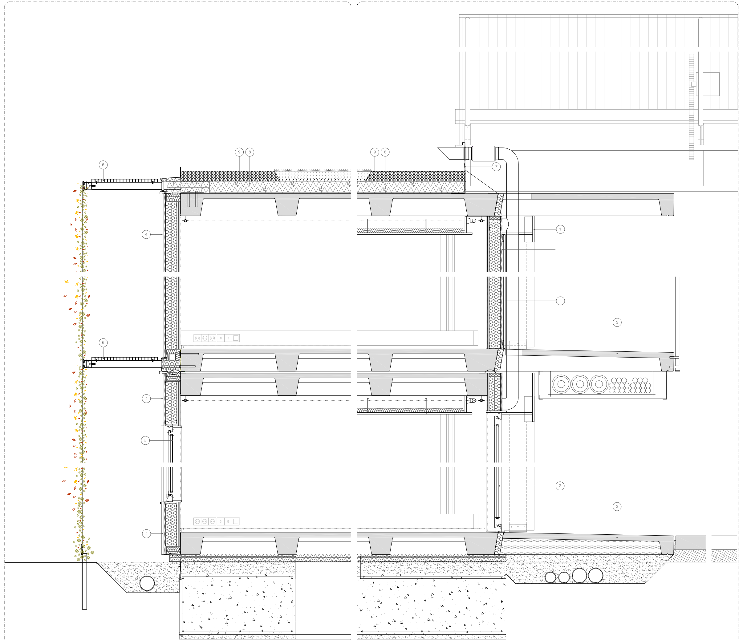
SECCIÓN CONSTRUCTIVA 0 0.2 1m
