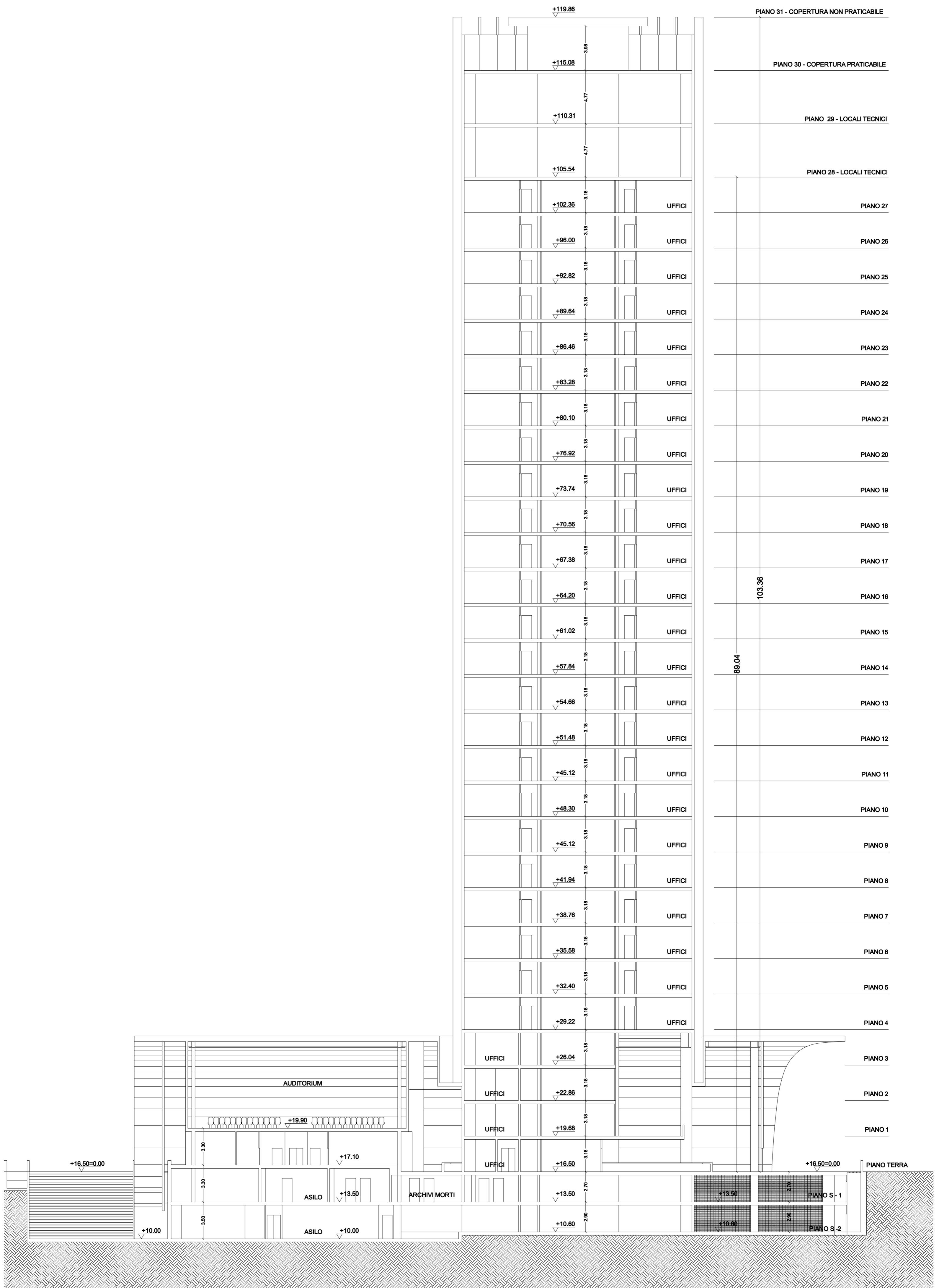
SEZIONE B-B
