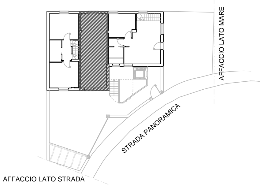
PIANO SEMINTERRATO (MQ. 35) (MQ. COMMERCIALI 25,12)
