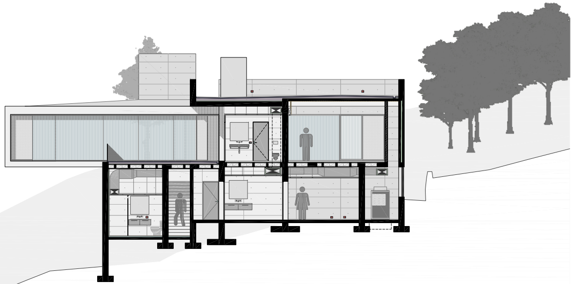
CORTE C
