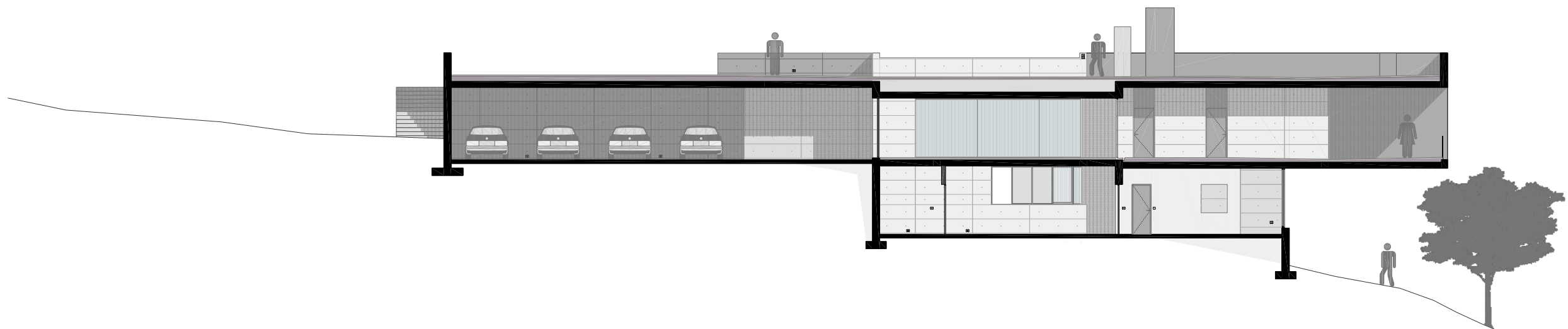
CORTE C
