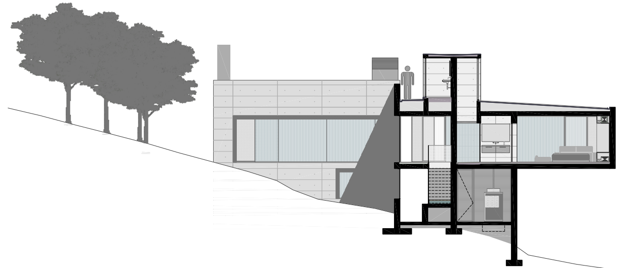
CORTE F
