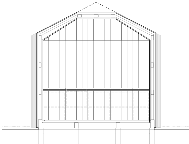
CORTE A
