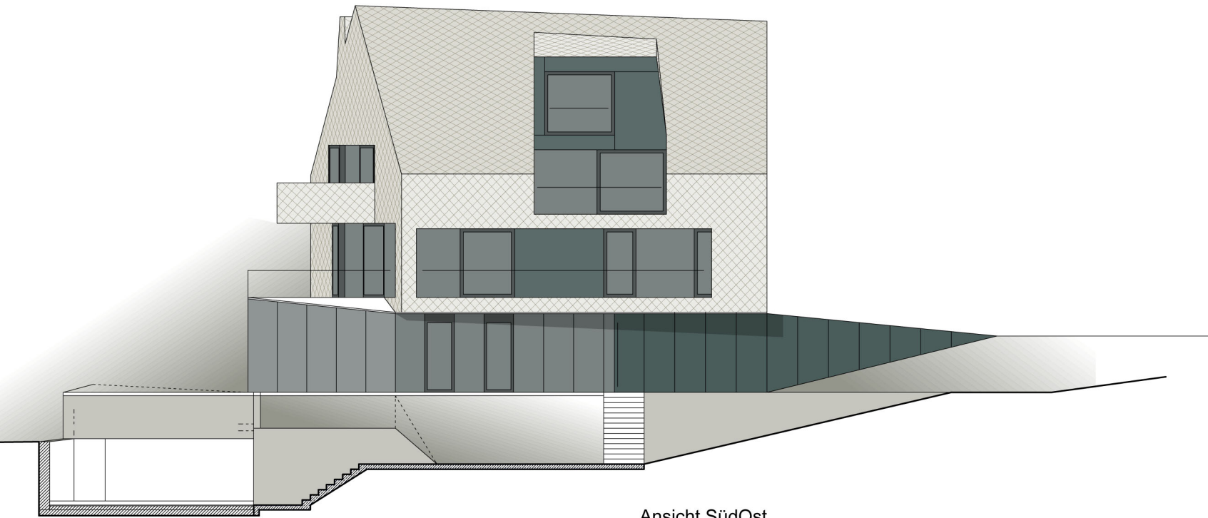
Ansicht SüdOst
