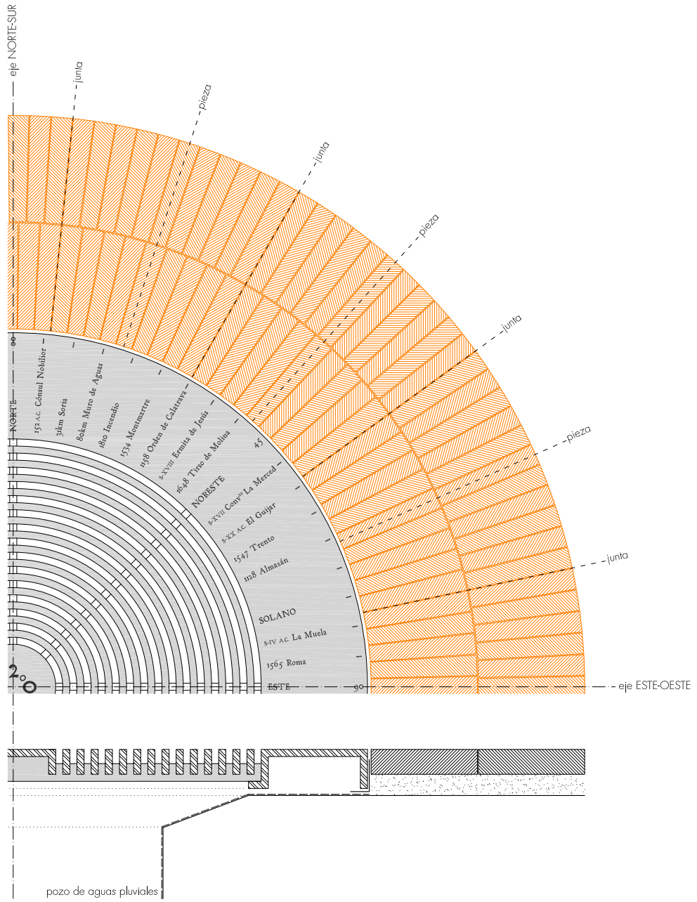
DETALLE ENCUENTRO REJILLA DE BRONCE CON PAVIMENTO CERÁMICO
