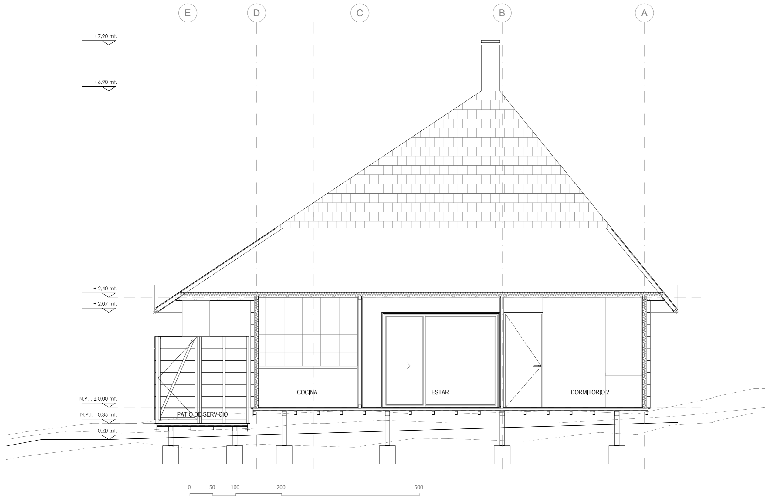
corte 1-1'
