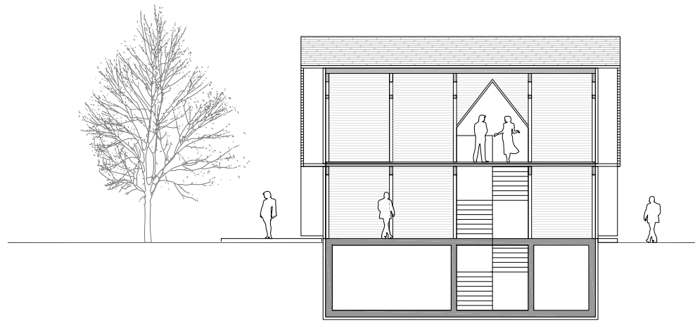
LÄNGSSCHNITT
