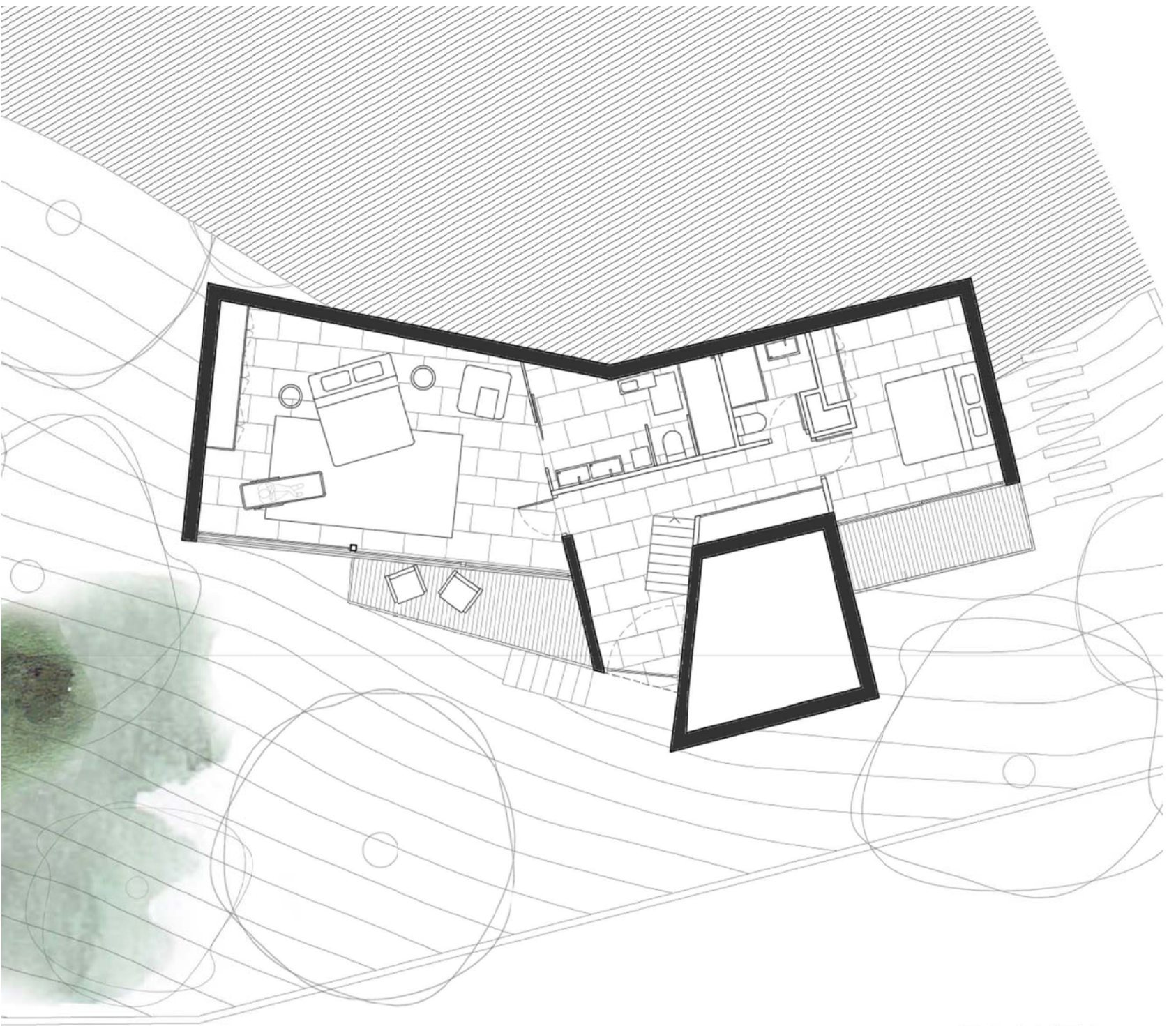
PLANTA -1
