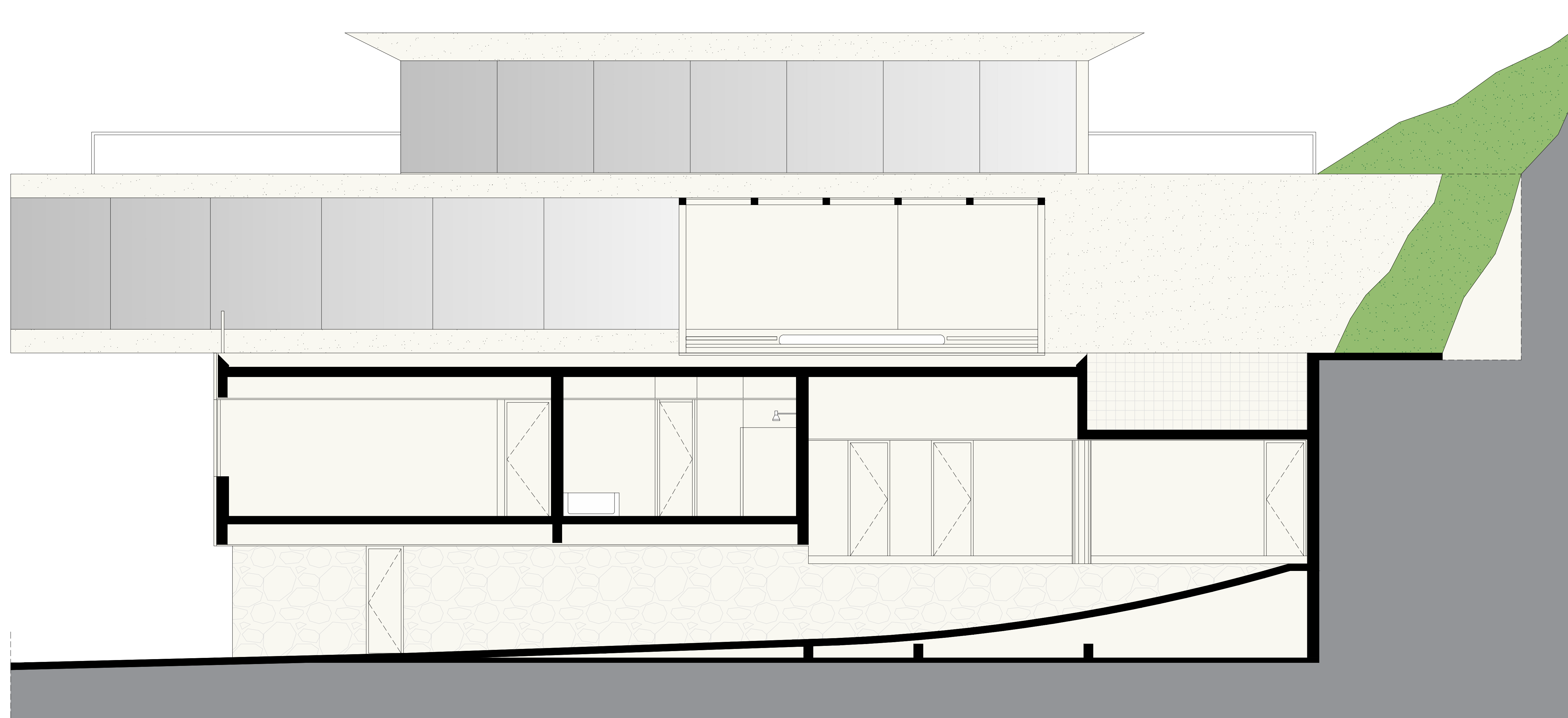
CORTE A
