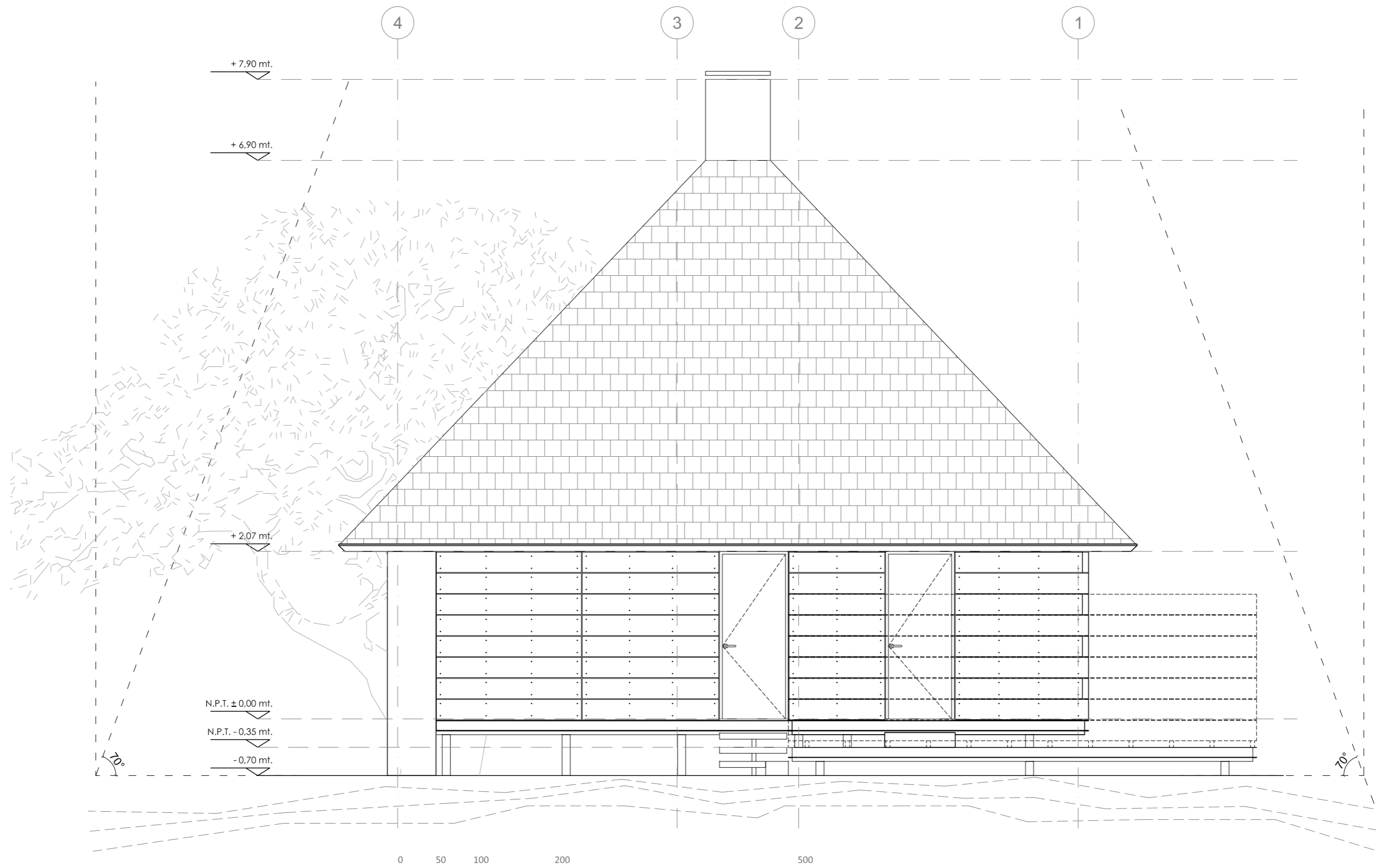
elevación sur
