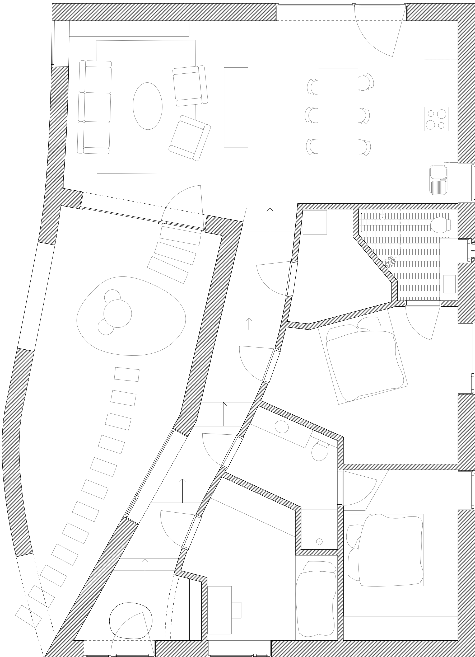
grondplan - schaal 1/50
