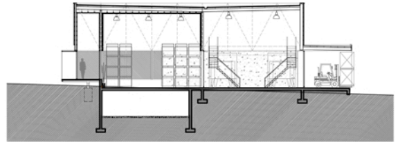
CORTE B.B
