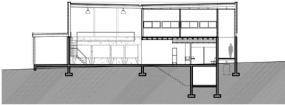
CORTE E.E
