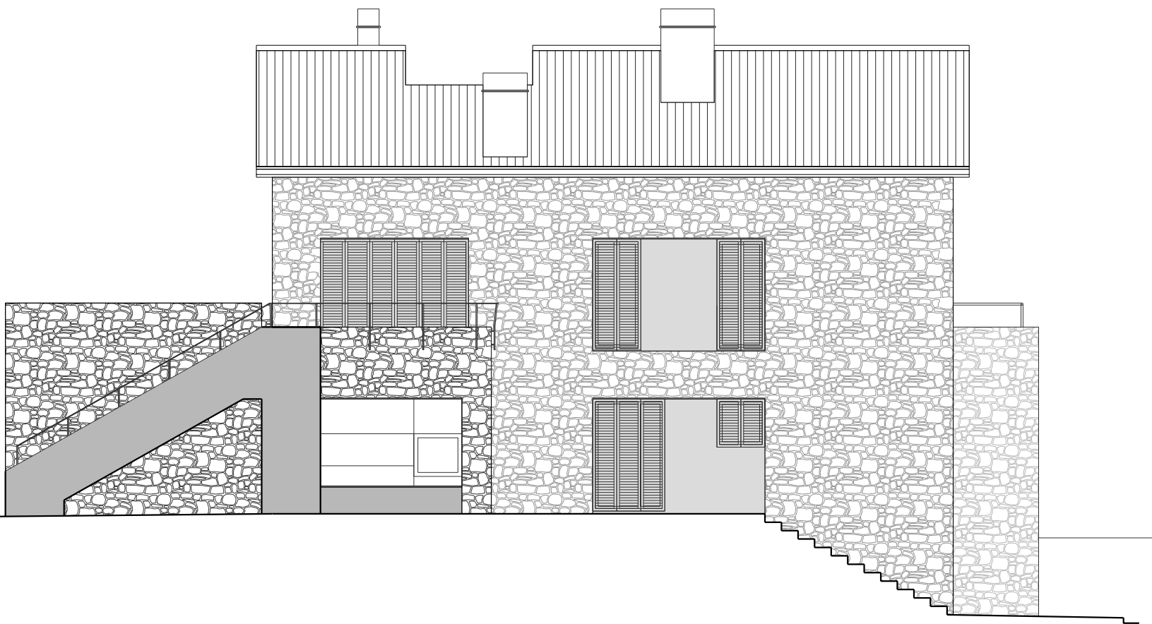
FAÇANA EST
