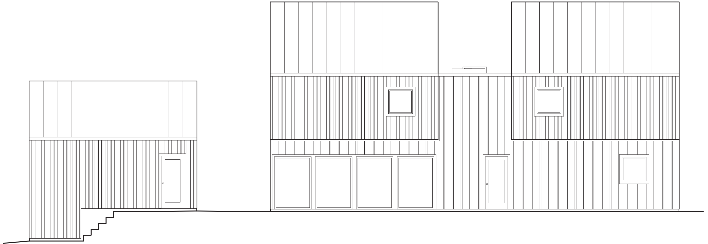
FACHADA SUR
