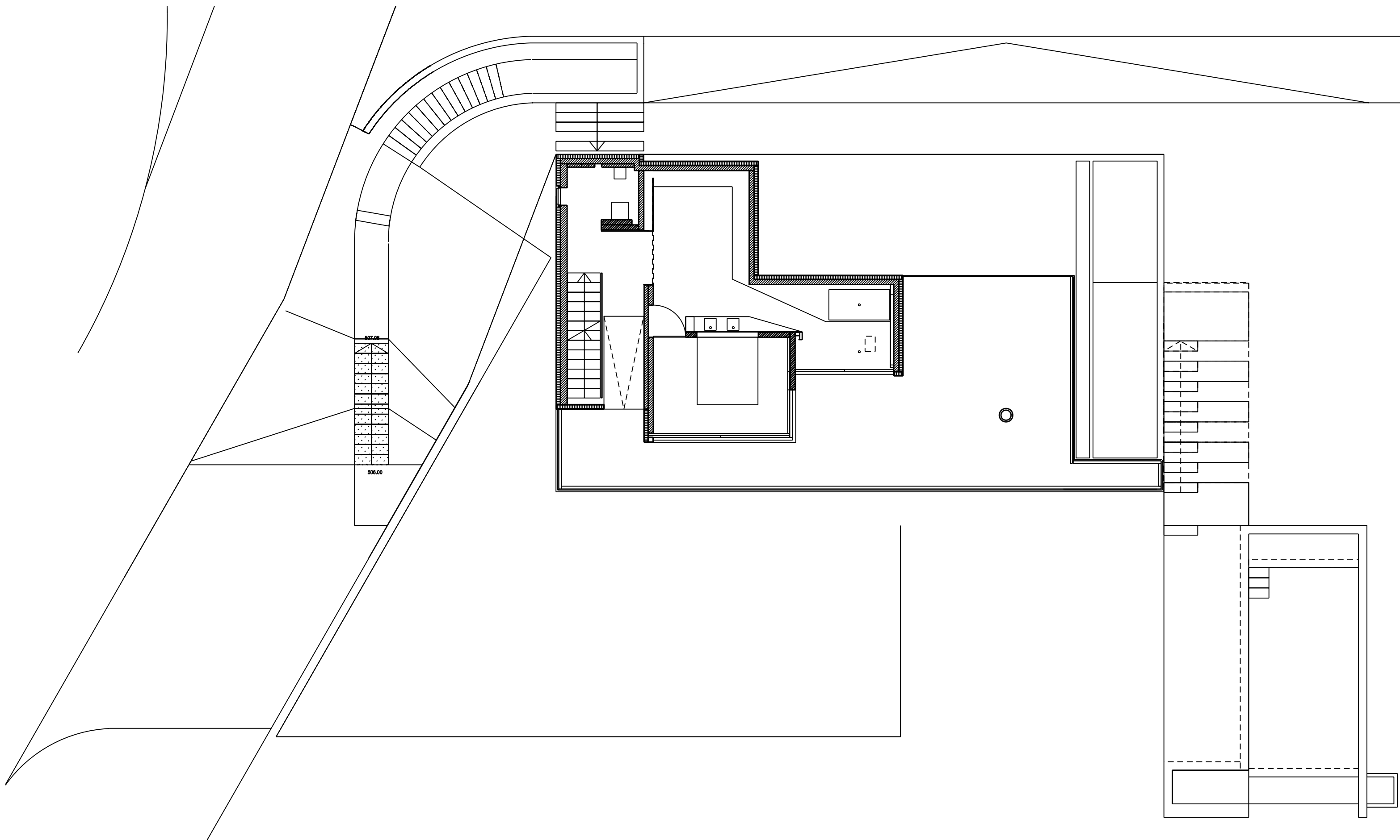
feldbalz house 1:100 lastfloor gus wüstemann ma eth sia coac
