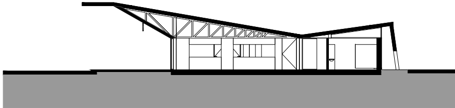
CORTE 01
