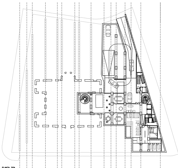
PLANTA SPA
