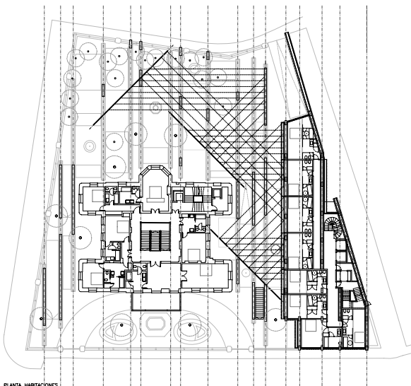
PLANTA HABITACIONES
