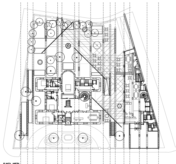
PLANTA JARDIN
