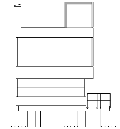
Nord-Fassade 0 1 2[m]
