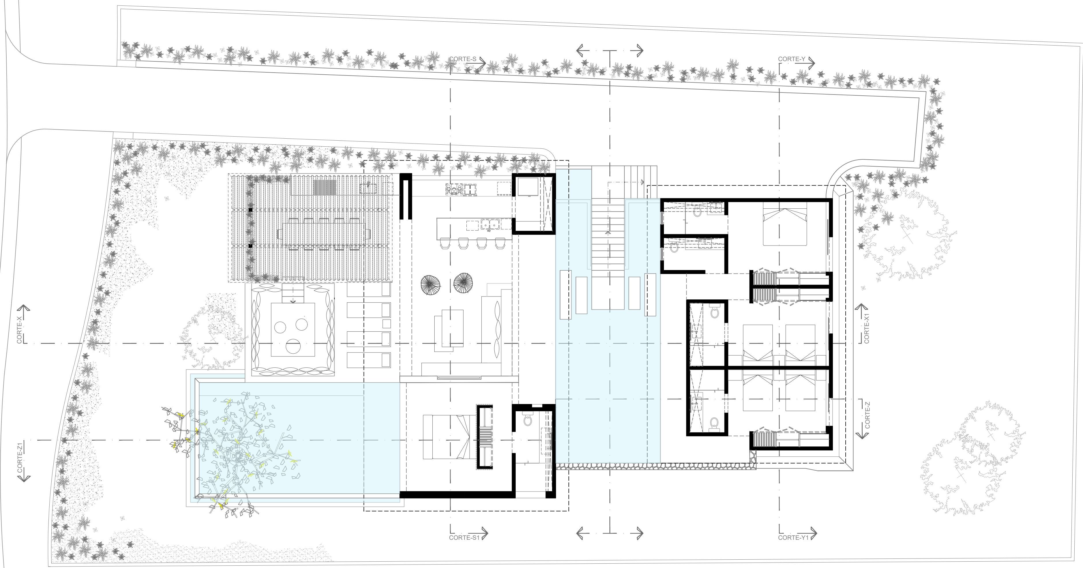
PLANTA ALTA
