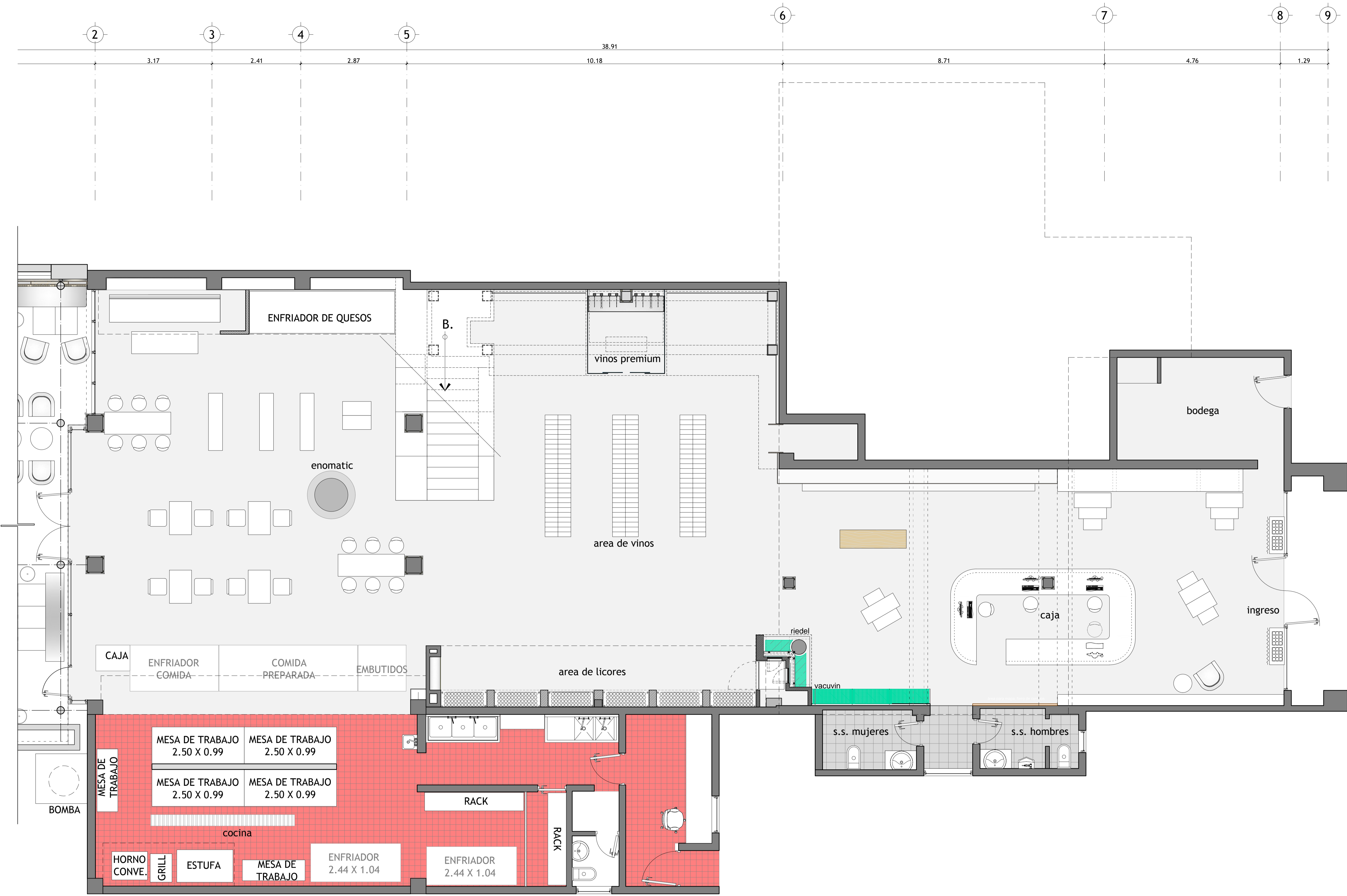
planta arquitectónica escala 1/50
