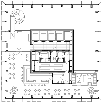
PLANTA PRIMERA / FIRST FLOOR PLAN
