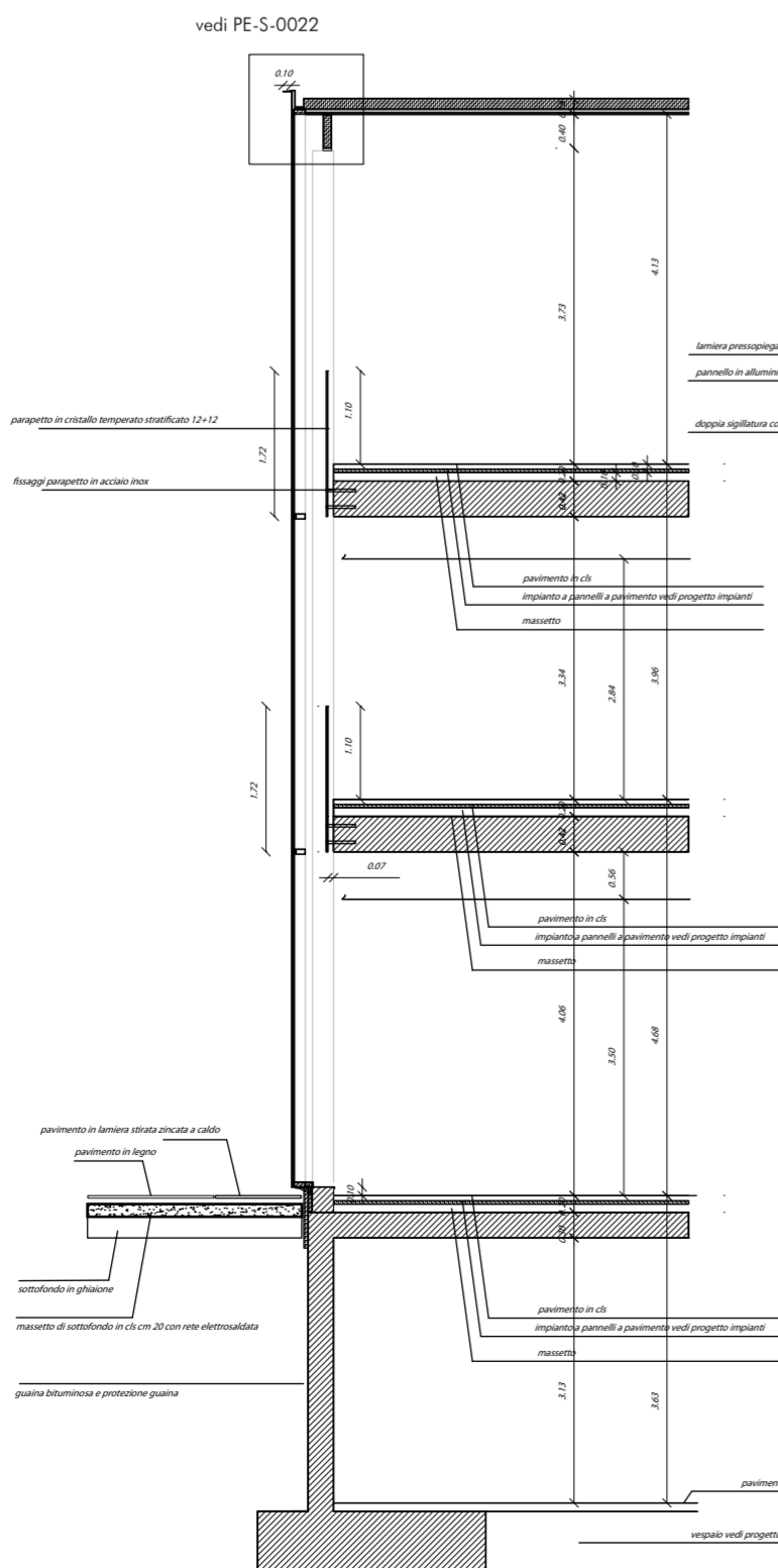
Dettaglio EE
