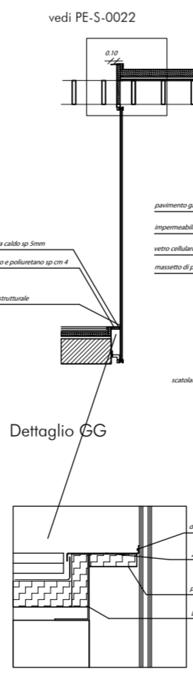
Dettaglio GG
