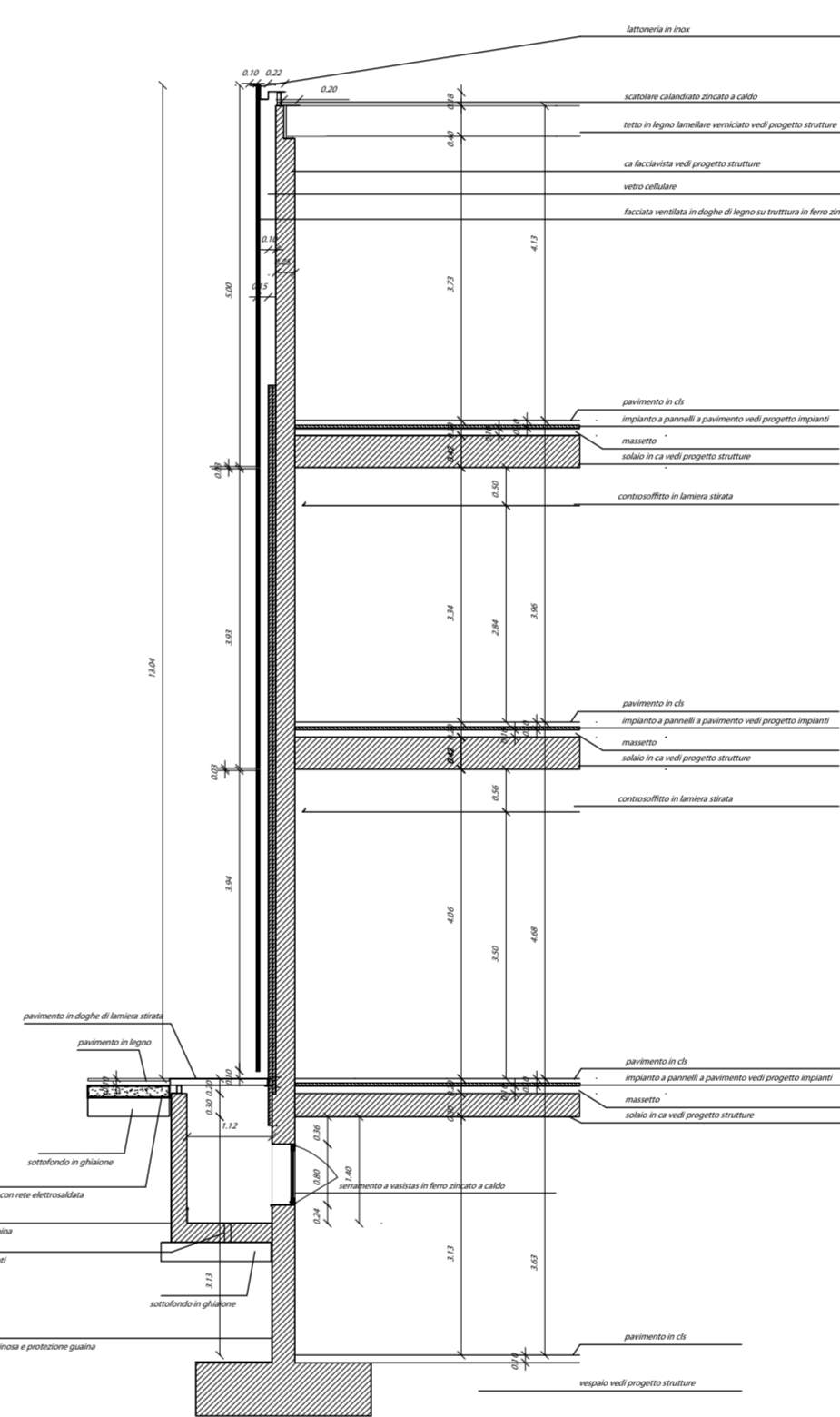
Dettaglio CC
