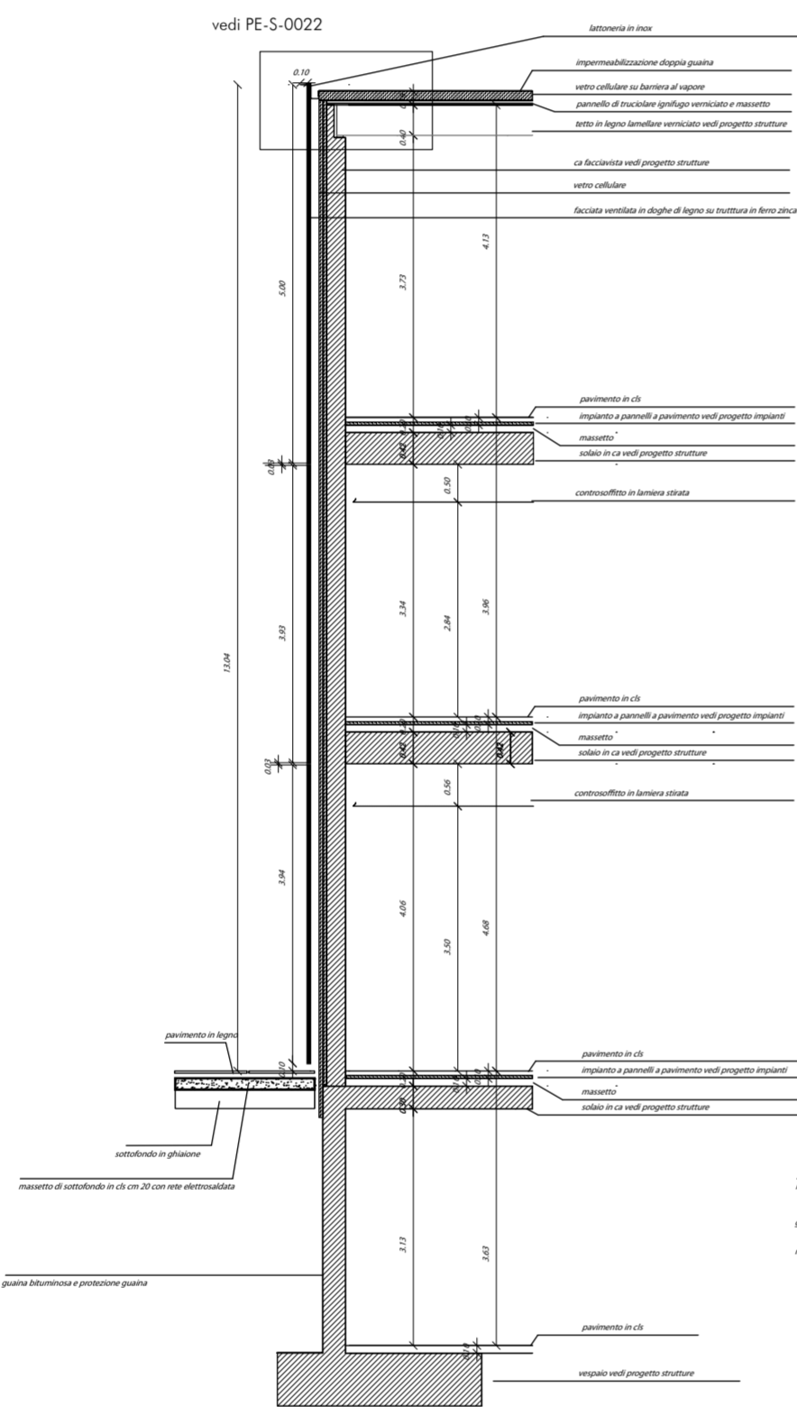
Dettaglio DD
