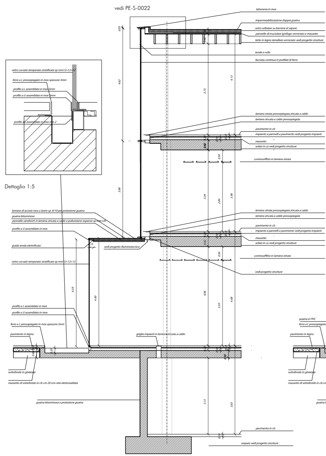
Dettaglio AA
