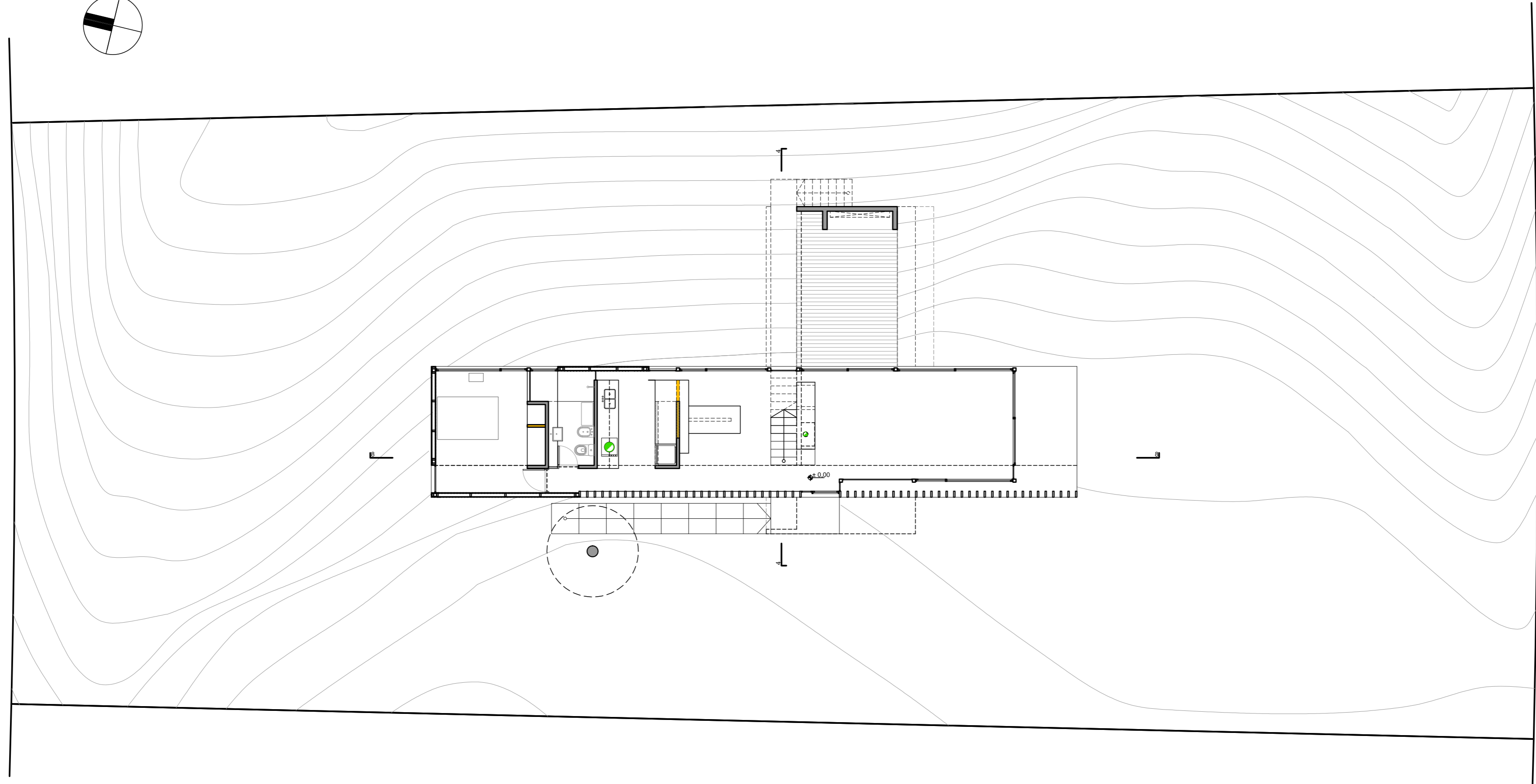
PLANTA BAJA
