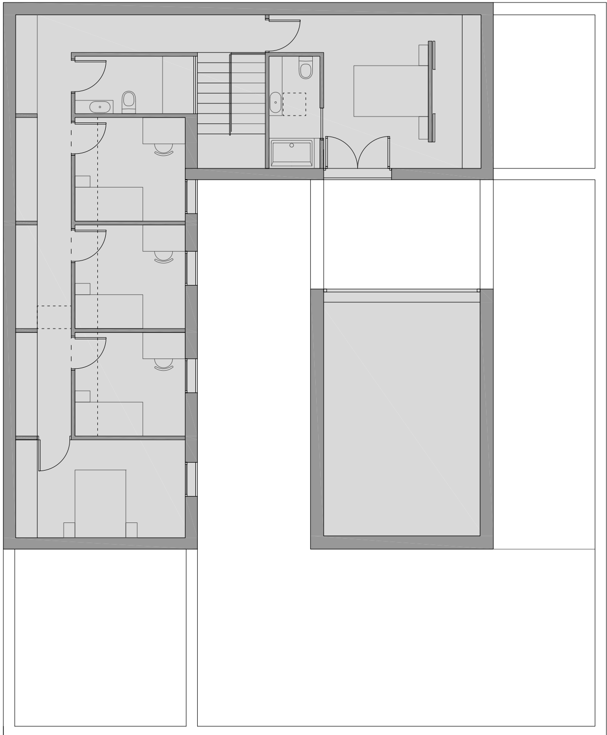
FIRST FLOOR PLANTA PRIMERA
