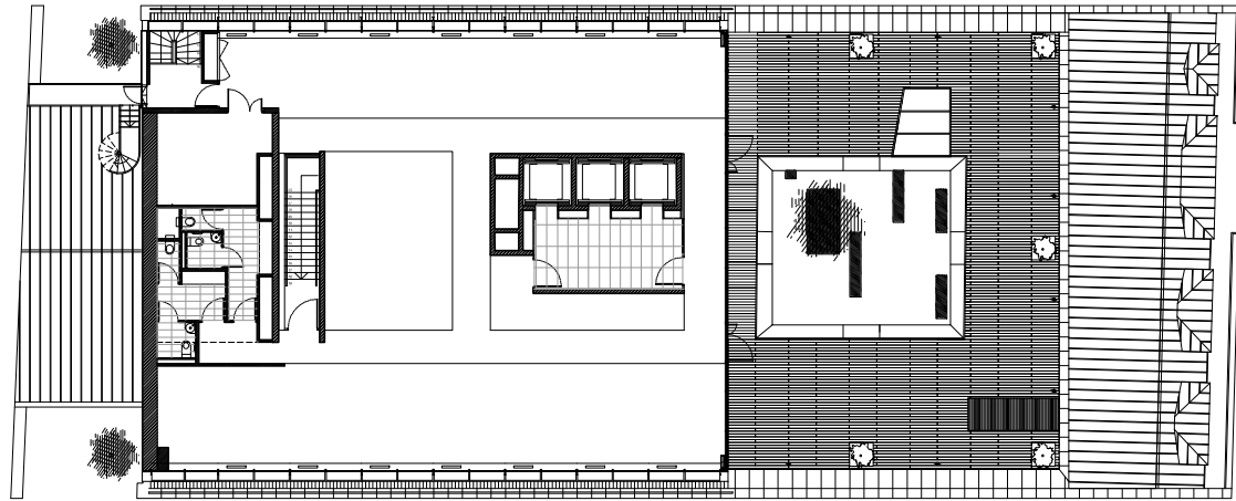
PLAN DE NIVEAU R+7 // ATELIERS 2/3/4/
