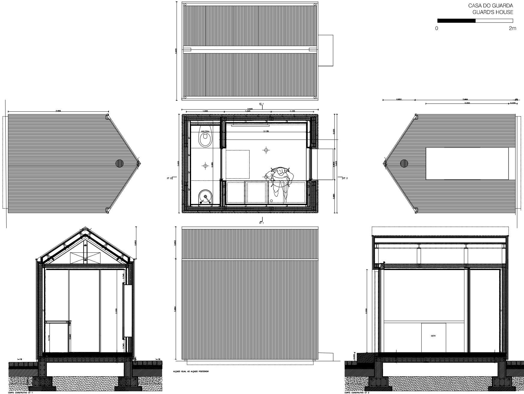
CORTE CONSTRUTIVO CT 1
