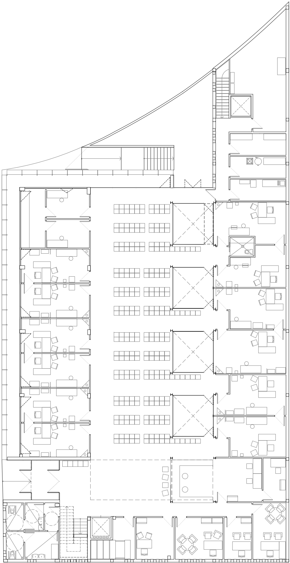
PLANTA BAJA
