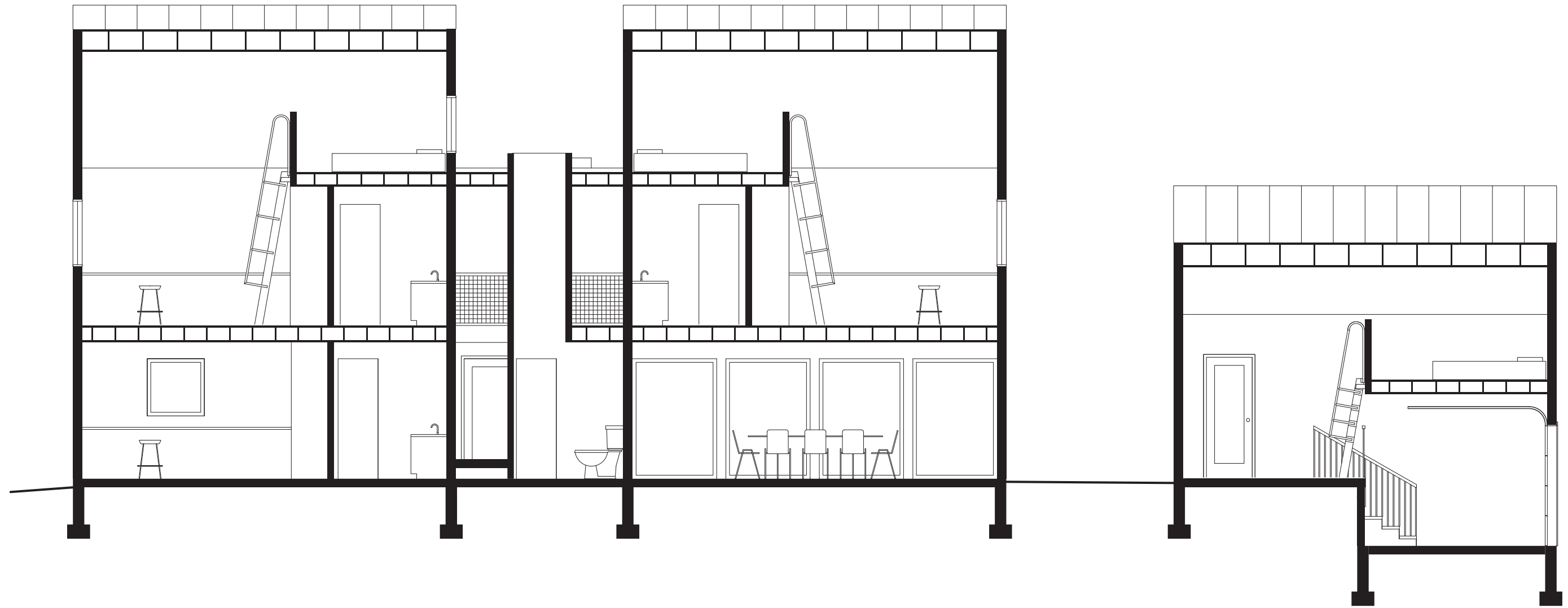
CORTE 1-1'
