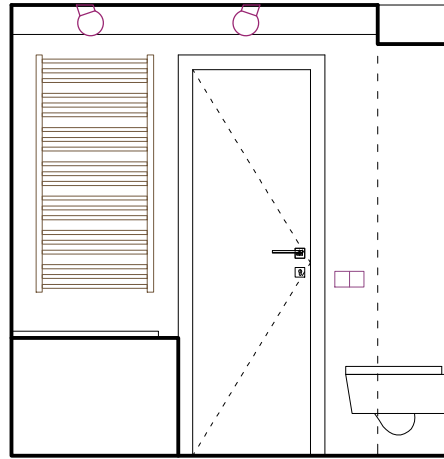
pohled A
