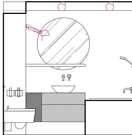
pohled B
