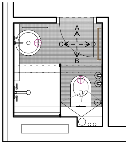
půdorys - malá koupelna
