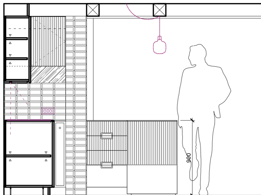
pohled C
