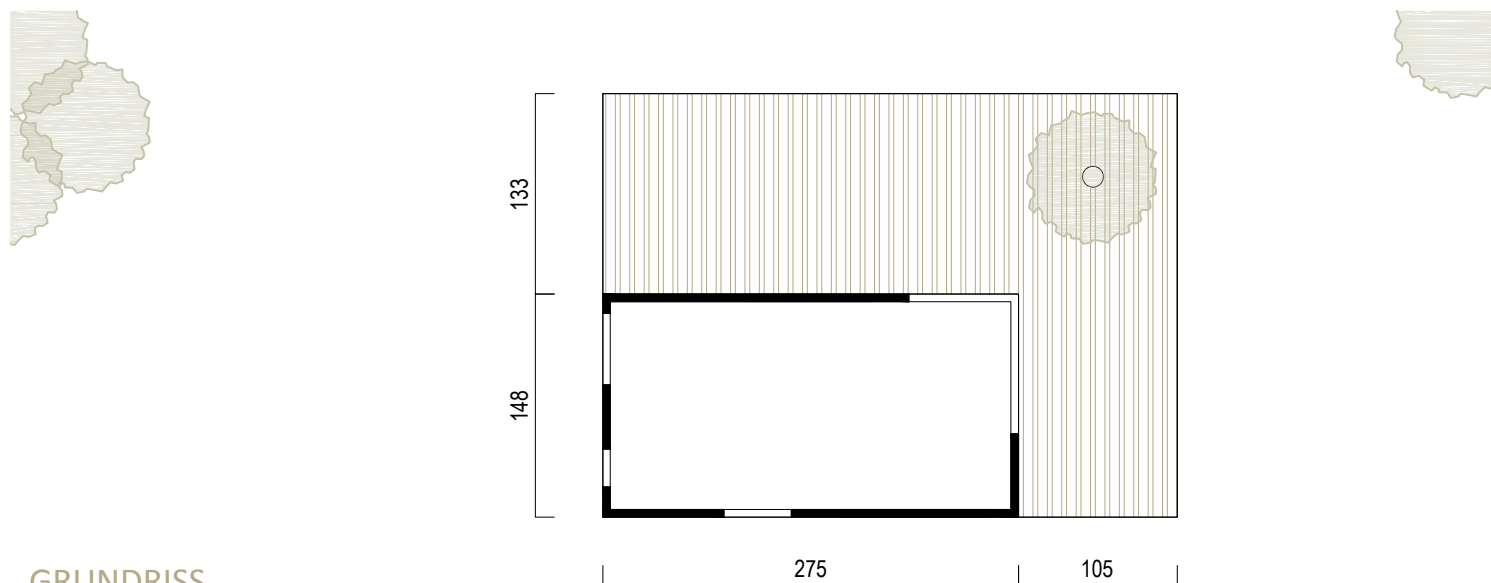
GRUNDRISS
