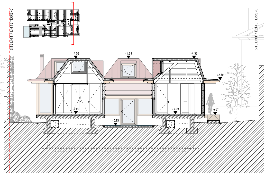
SECTION 5 CORTE 5
