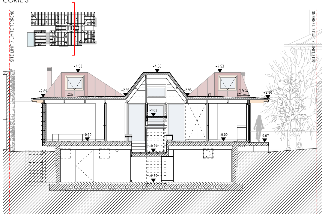
SECTION 4 CORTE 4
