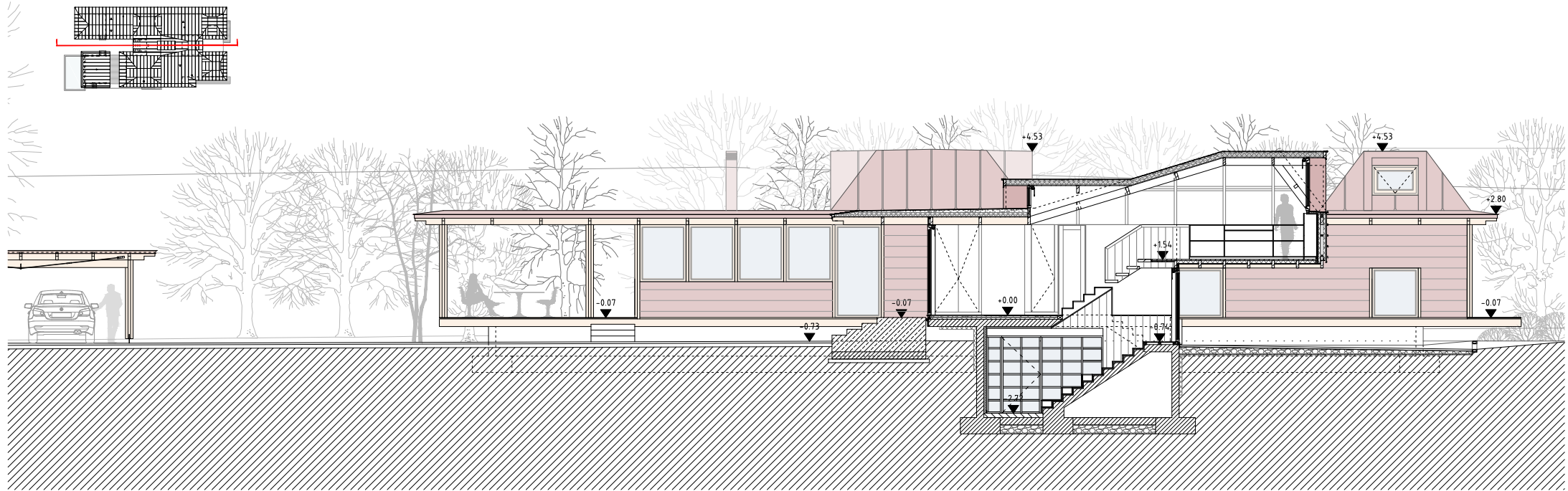
SECTION 1 CORTE 1
