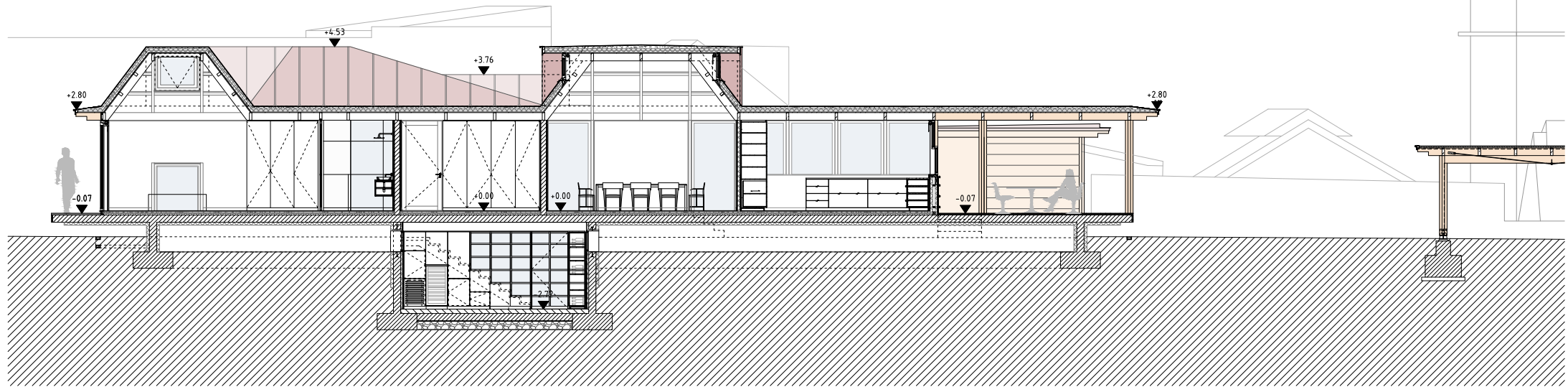
SECTION 3 CORTE 3
