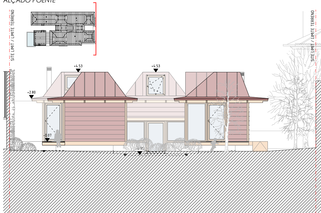
NORTH ELEVATION ALÇADO NORTE
