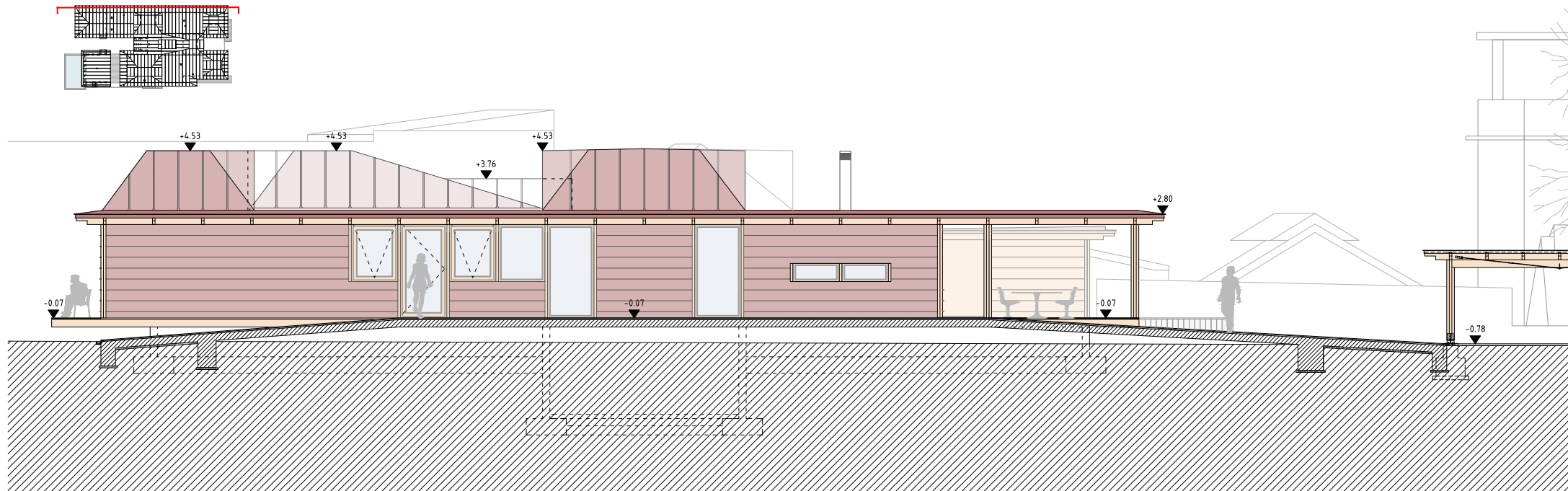
WEST ELEVATION ALÇADO POENTE
