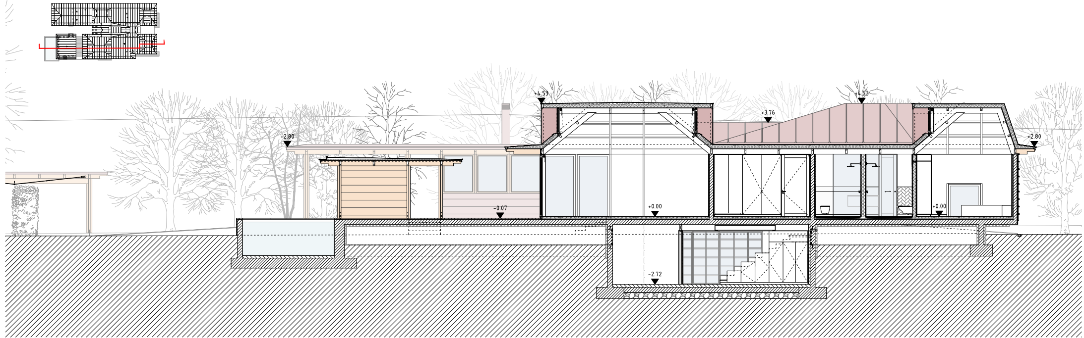
SECTION 2 CORTE 2
