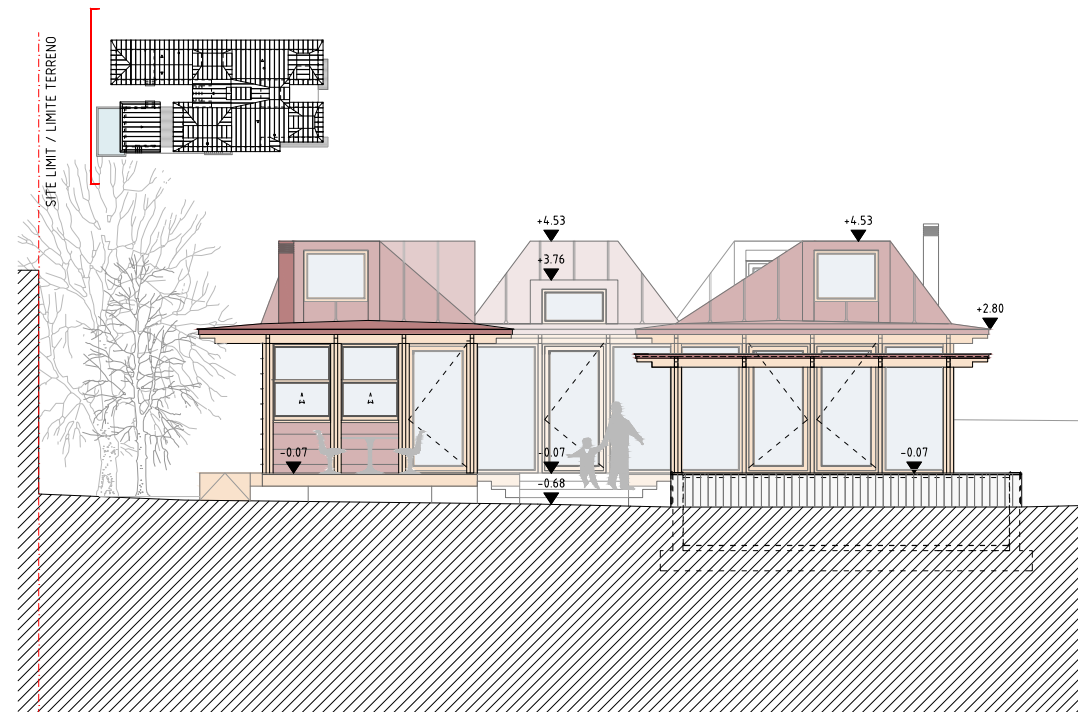
SOUTH ELEVATION ALÇADO SUL
