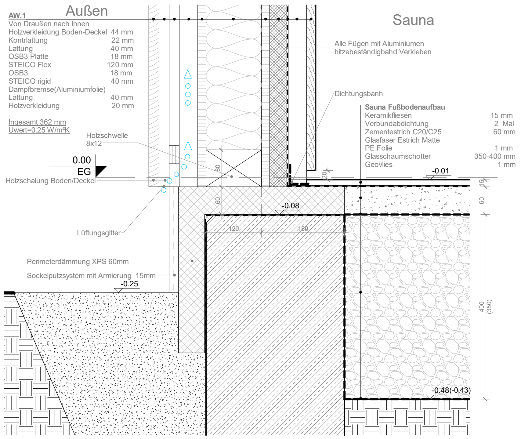
Det 302 Sockelanschluss und Bodenaufbau Sauna.
