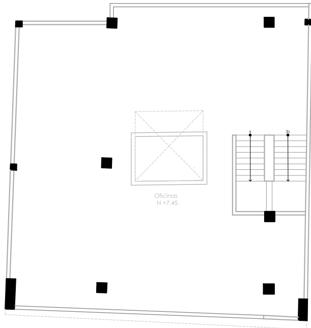
NIVEL 3
