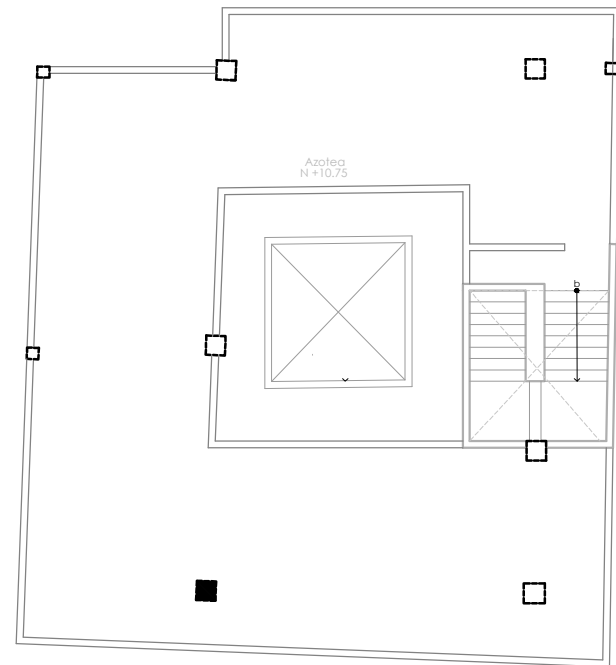
NIVEL AZOTEA
