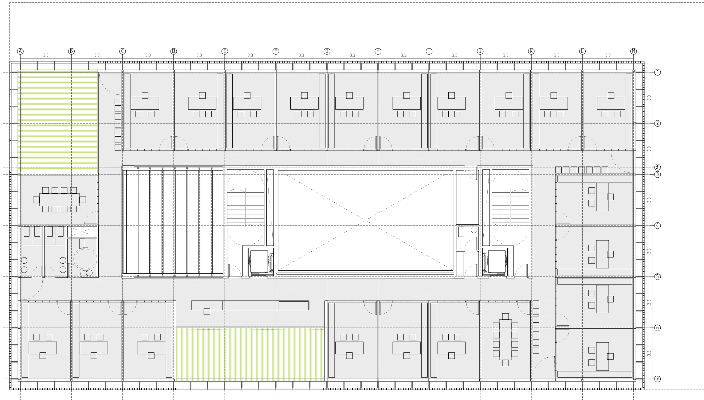
E 1:150 PLANTA PRIMERA
